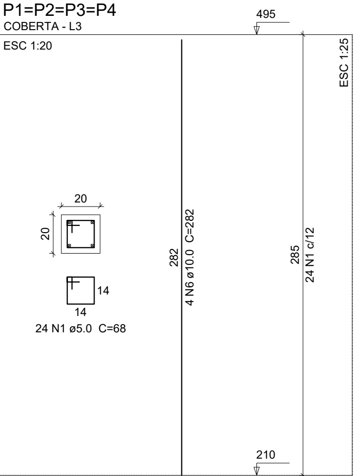
Detalhe Pilares – Caldeira escala →
