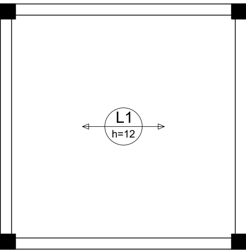
Armação Positiva (eixo X) – Caldeira escala → 1/50
