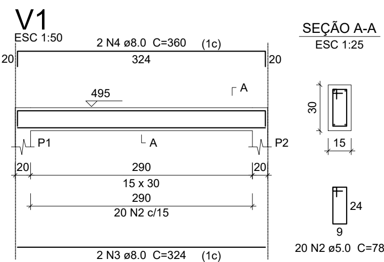
Detalhe Vigas – Caldeira escala →
