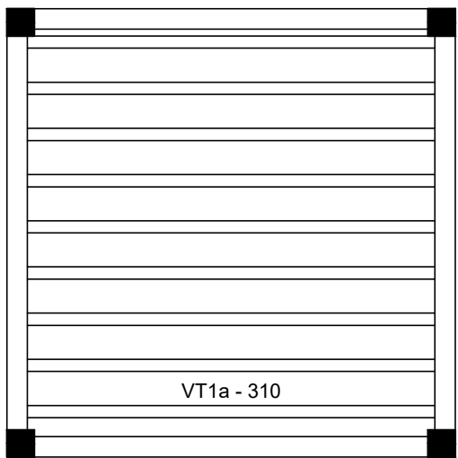
Planta Vigotas pré-moldadas – Caldeira escala → 1/50
