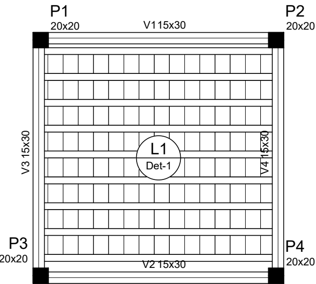
Forma Coberta – Caldeira escala → 1/50
