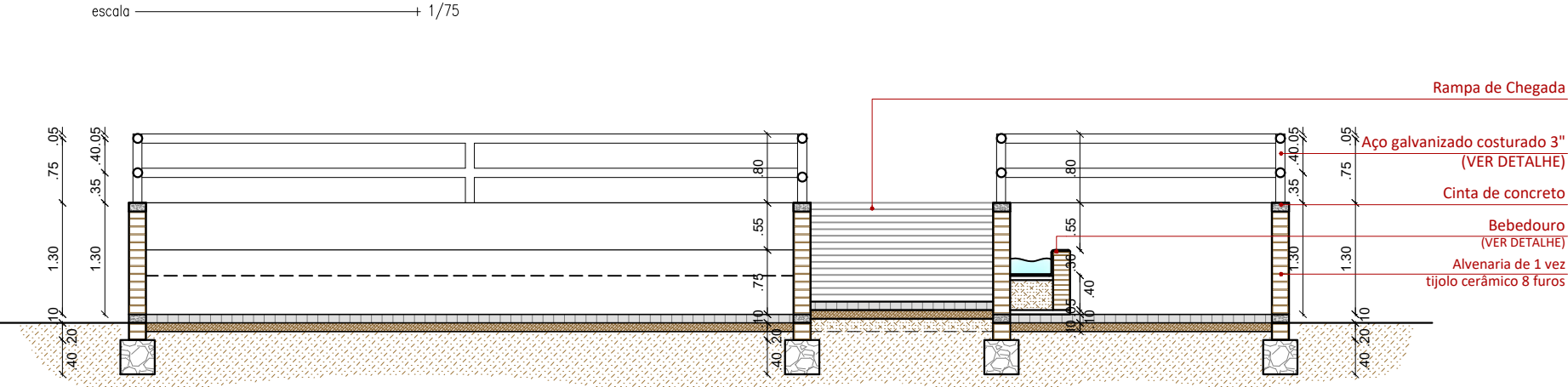
Corte BB – Curral Bovino
