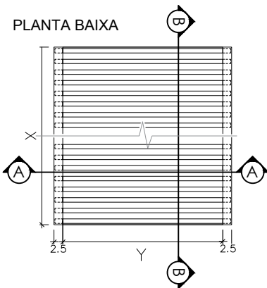
Detalhe – Canaleta com Grelha escala + 1/15
