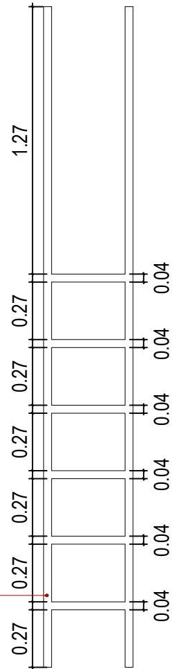
Escada Marinheiro 02 Plataforma de Observação
