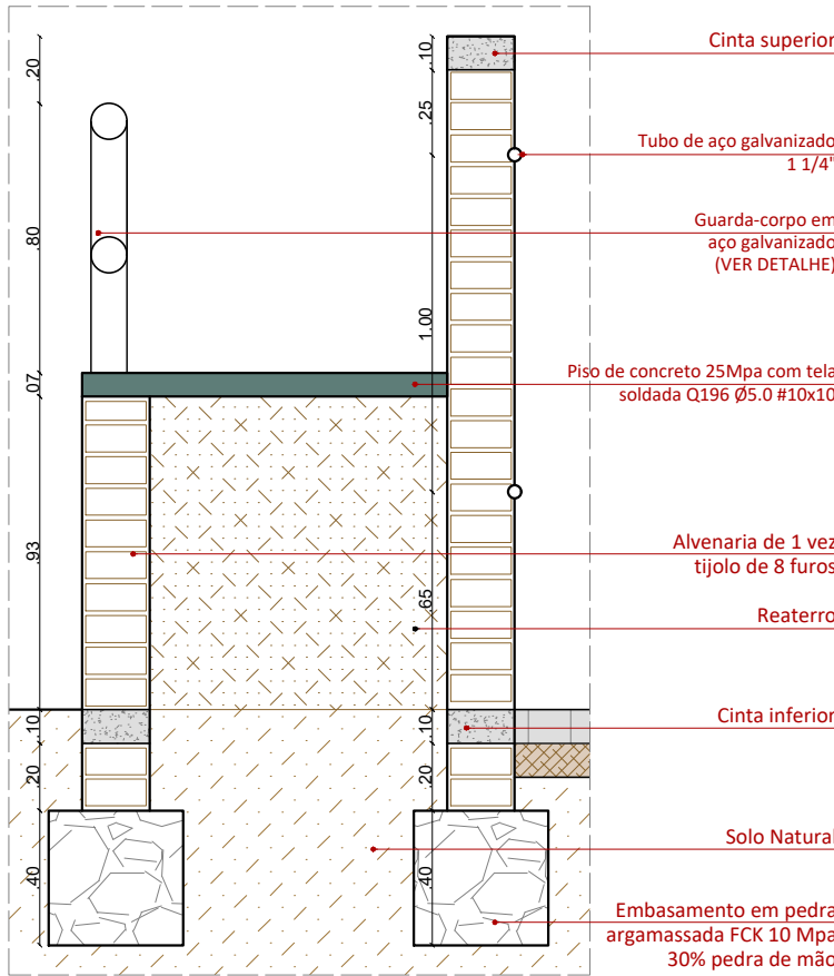
Detalhe – Plataforma escala + 1/25
