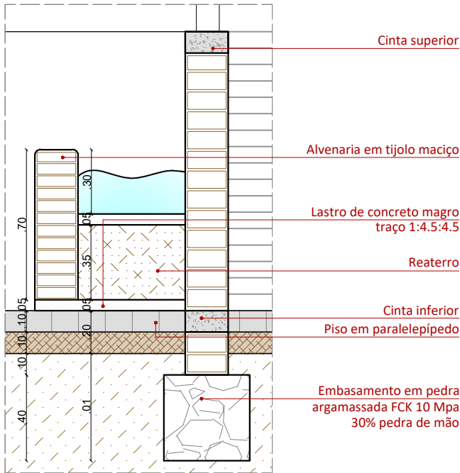
Detalhe – Bebedouro escala + 1/25
