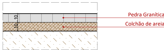
Detalhe – Piso paralelepípedo escala + 1/25
