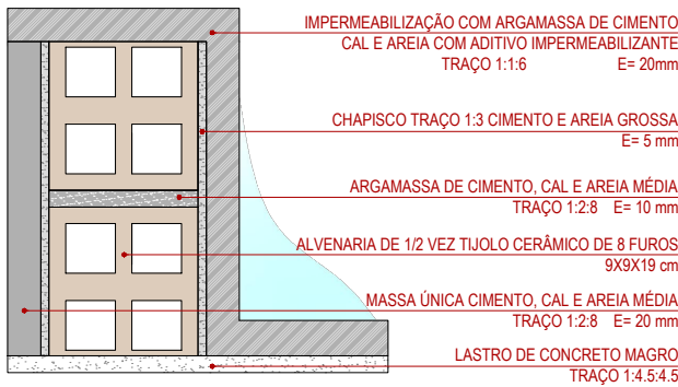
Detalhe – Bebedouro escala + 1/5
