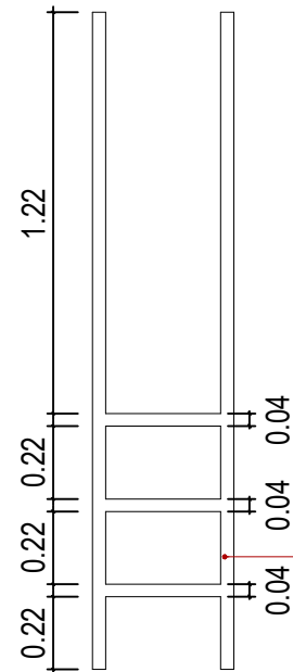
Escada Marinheiro 01 Plataforma do Marteleiro
