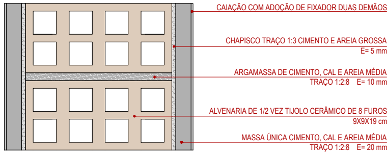
Detalhe – Alvenaria Geral escala + 1/5
