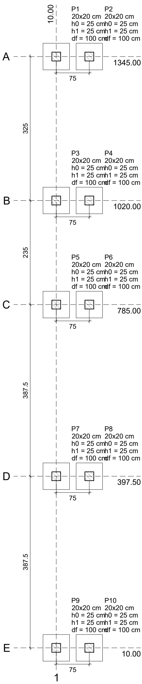
Locação Fundação – Curral bovino escala 1/50
