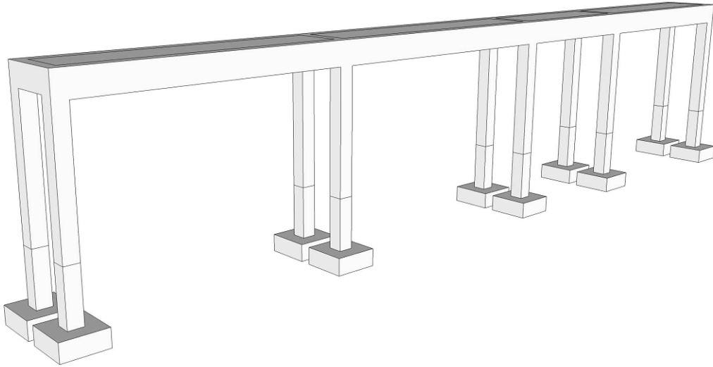
Maquete Estrutural 3D – Plataforma de observação do Curral Bovino escala 1/50
