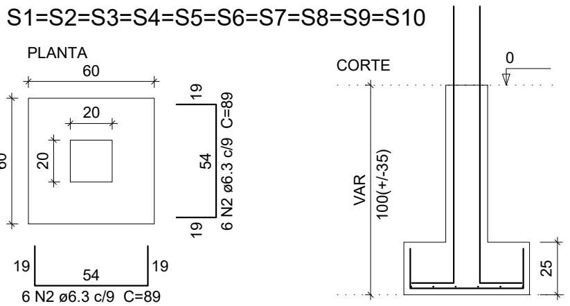
Detalhe Fundação – Curral bovino
