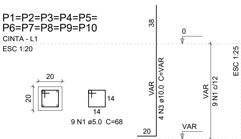
Detalhe Pilares – Curral bovino
