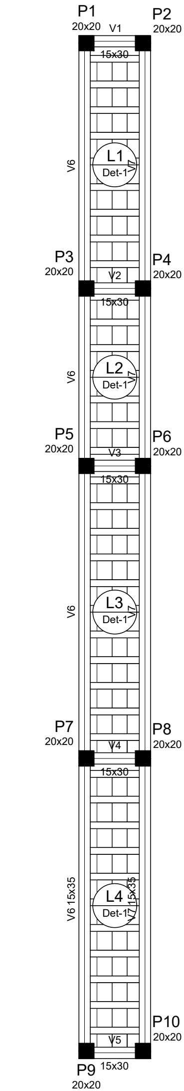
Forma da Plataforma – Curral bovino escala 1/50
