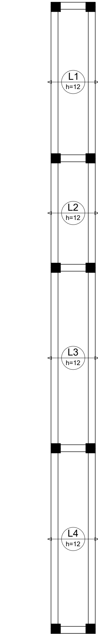
Armação positiva (eixo X) da Plataforma – Curral bovino escala 1/50
