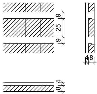
Detalhe laje – Curral bovino escala 1/50
