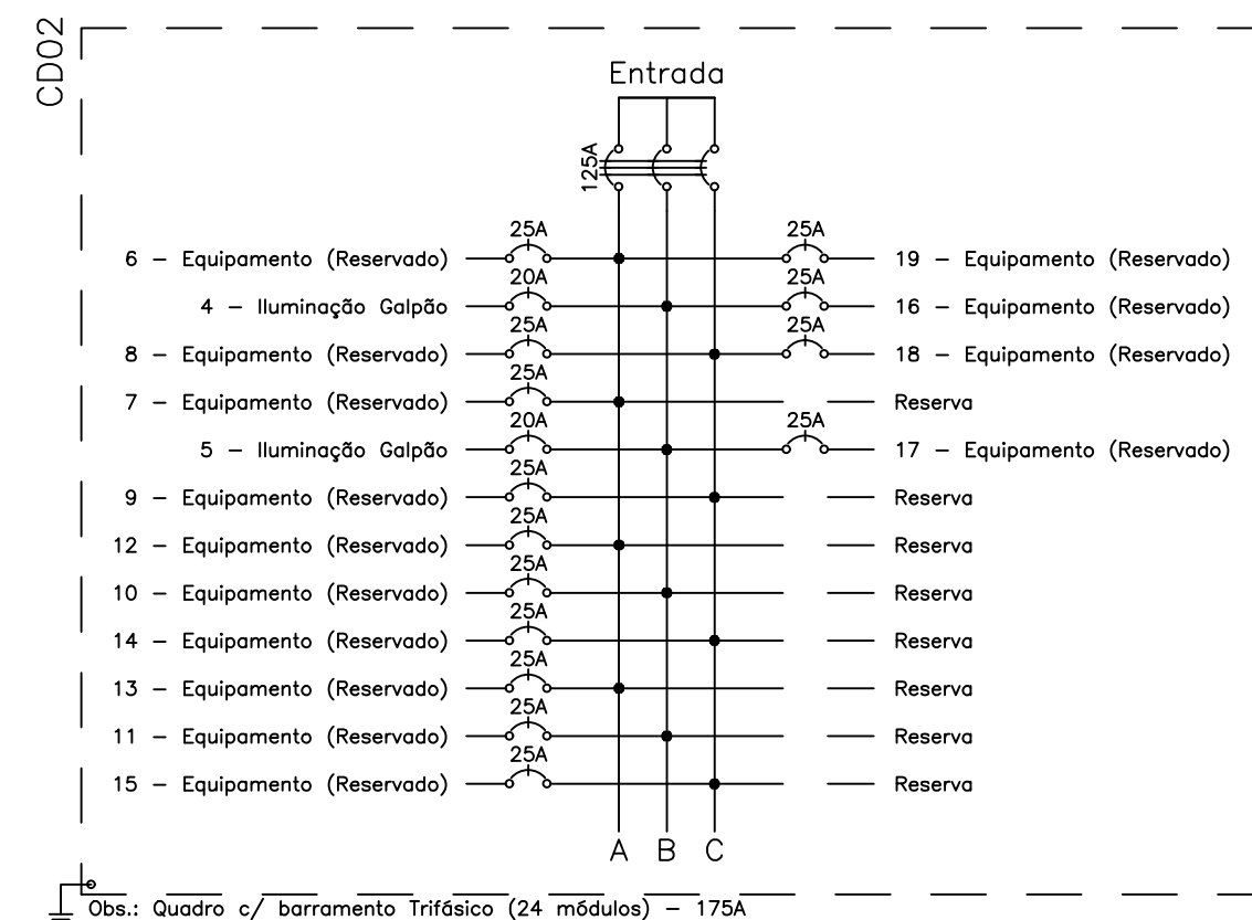
Obs.: Quadro c/ barramento trifásico (24 módulos) - 175A
