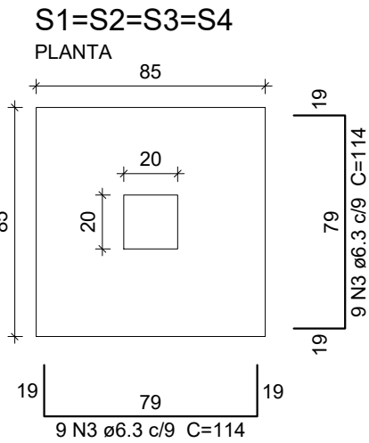
Detalhe Fundação – Sala de Painéis
