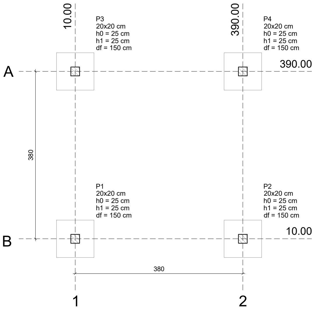
Localização estrutural – Sala de Painéis
