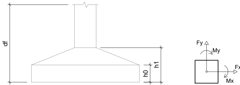
Detalhe estrutural – Sala de Painéis
