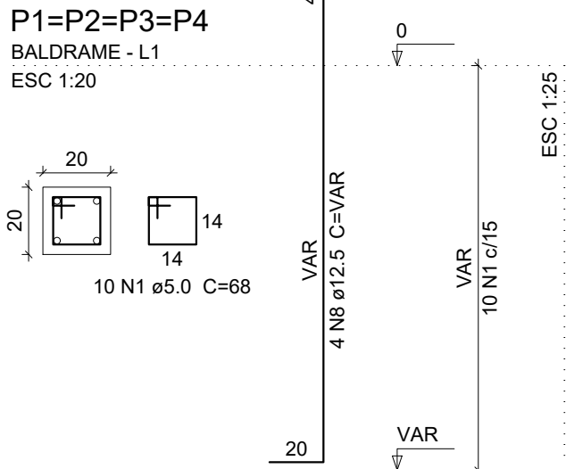
Detalhe Pilares – Sala de Painéis
