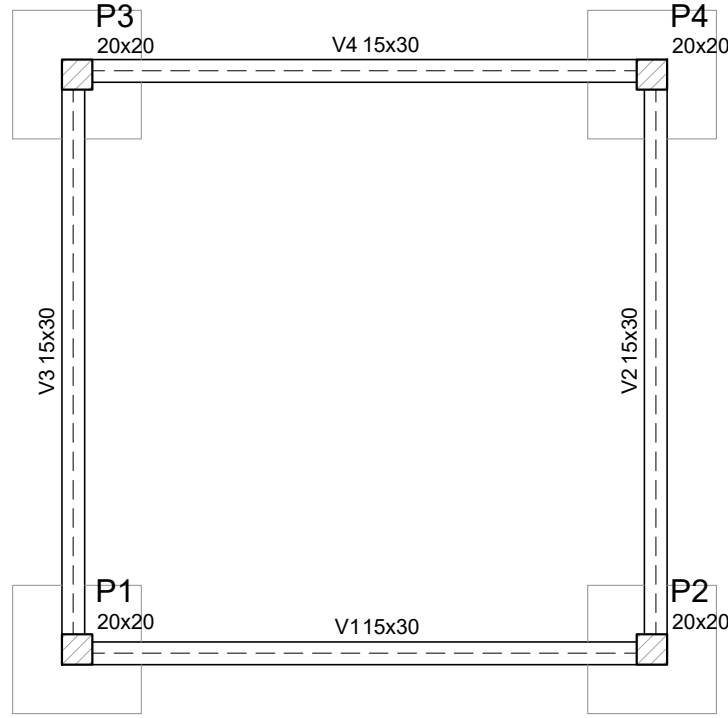
Forma Baldrame – Sala de Painéis
