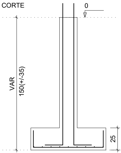
Detalhe Fundação – Sala de Painéis
