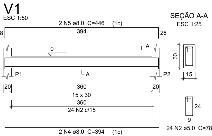
Detalhe Fundação – Vigas
