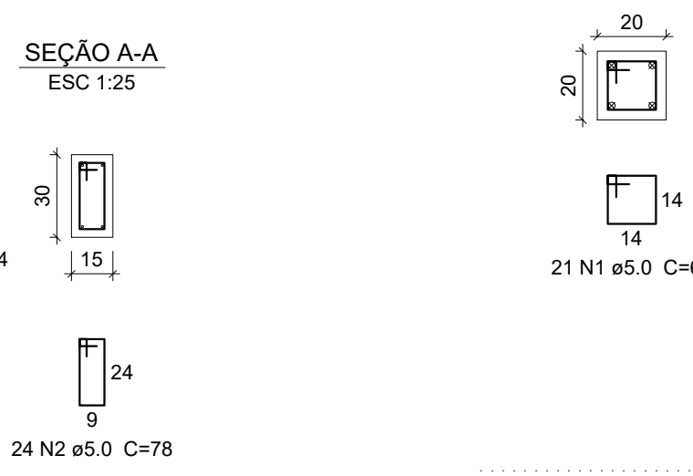
Detalhe Pilares – Casa de Máquinas escala →
