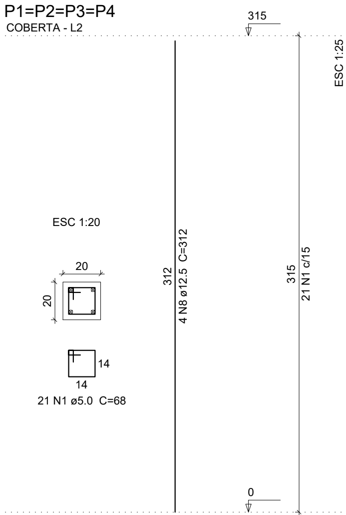
Detalhe Pilares – Casa de Máquinas escala →
