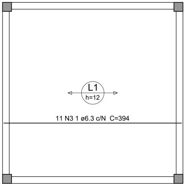
Armação Positiva (eixo X) – Casa de Máquinas escala → 1/50
