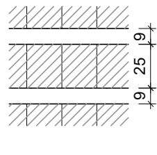
Detalhe – laje treliçada escala → 1/30
