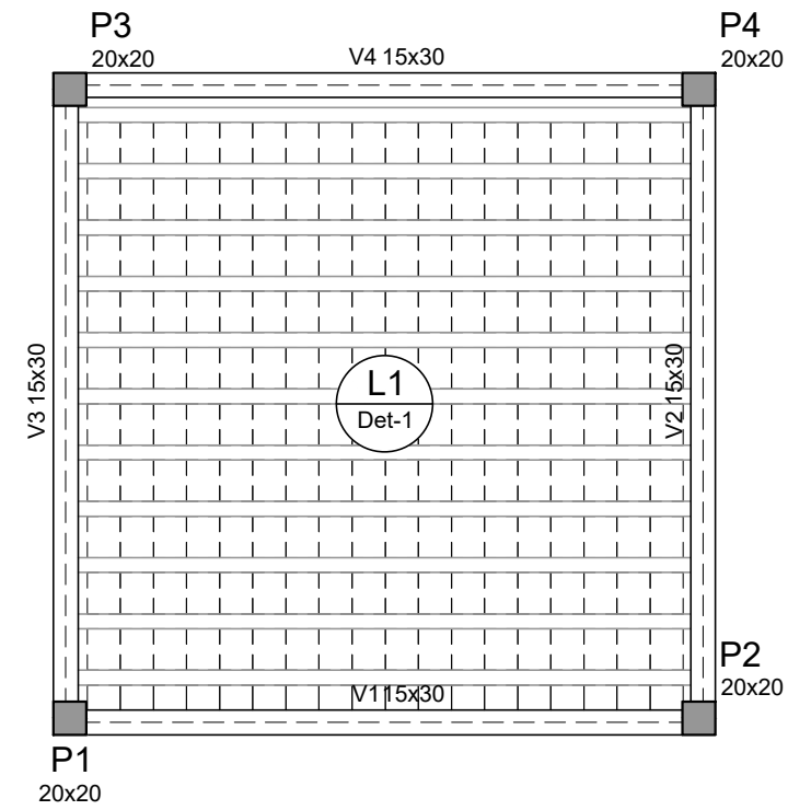
Forma Coberta – Casa de Máquinas escala → 1/50
