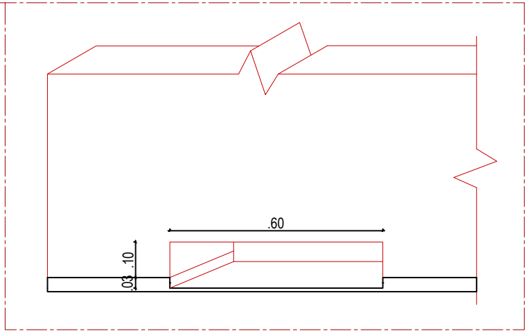
Detalhe – passagem sob paredes escala 1/15
