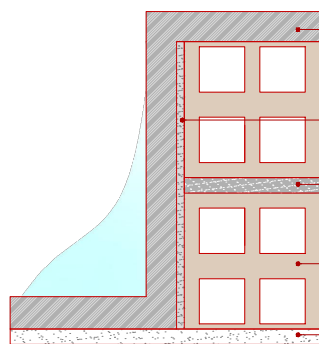
Detalhe – Grelha escala 1/5
