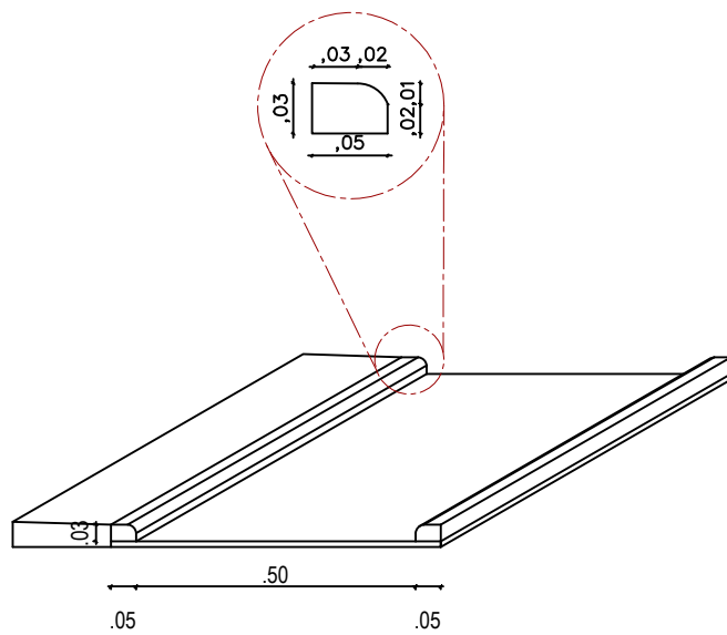
Detalhe – Canaleta escala 1/10
