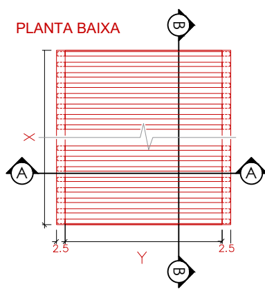
Detalhe – Grelha de drenagem escala 1/15
