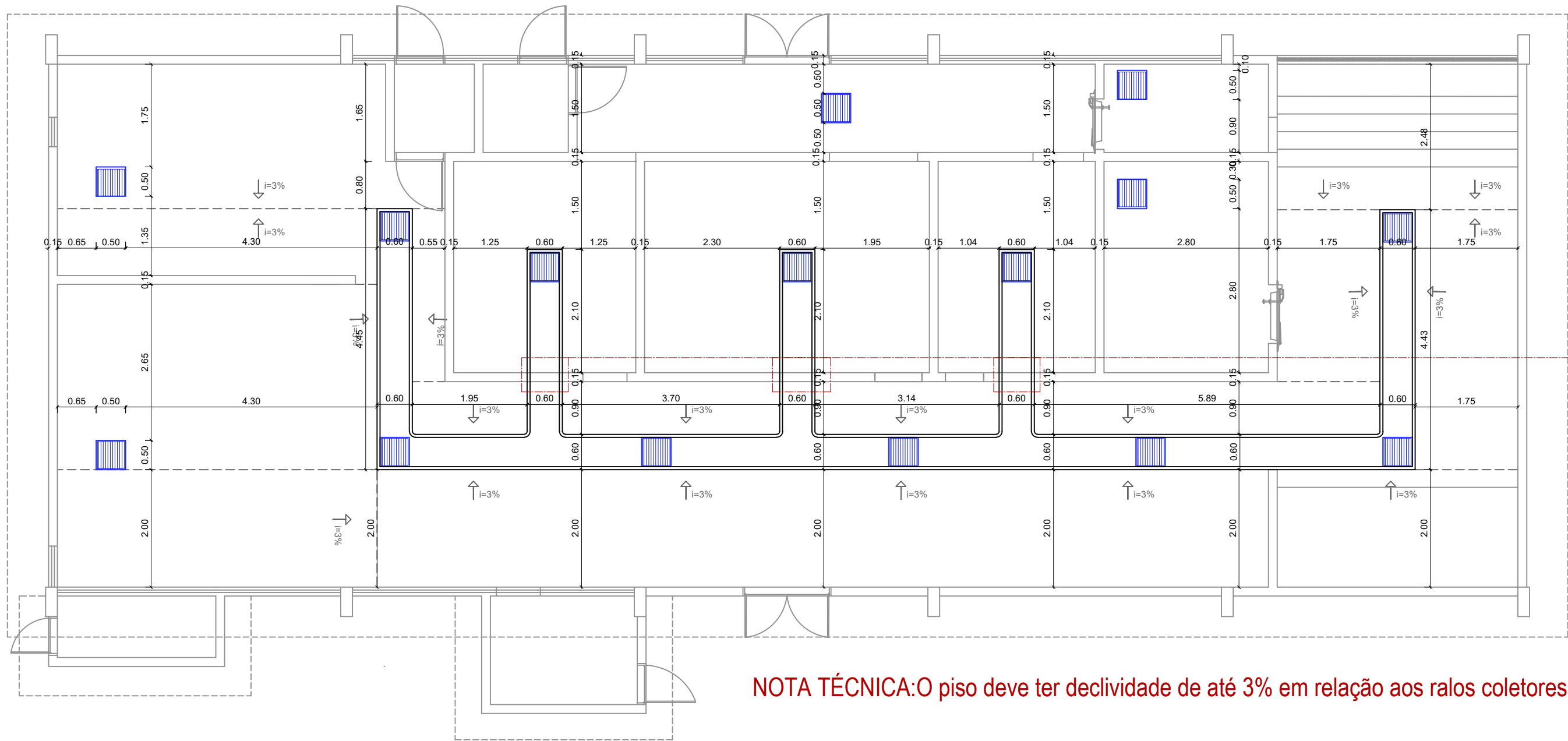
Planta Baixa Canaletas – Galpão escala 1/75
