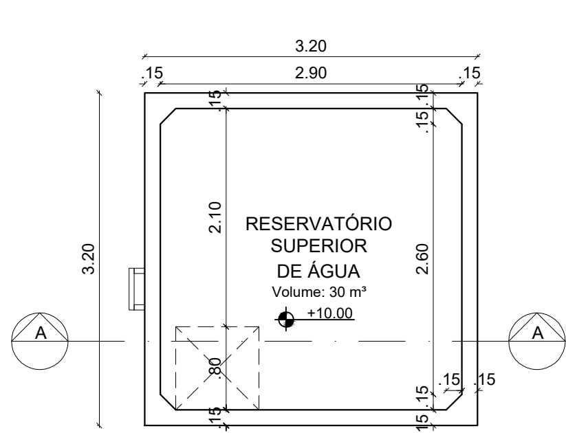
Planta Baixa – Reservatório Superior escala 1/50
