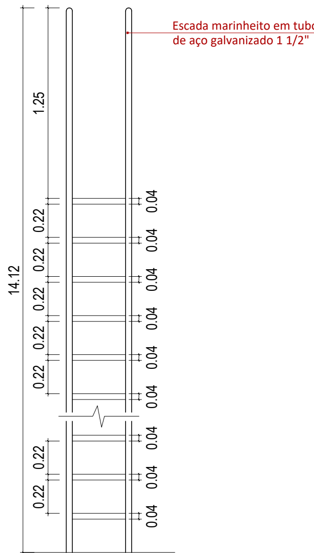
Detalhes – Escada Marinheiro escala 1/25
