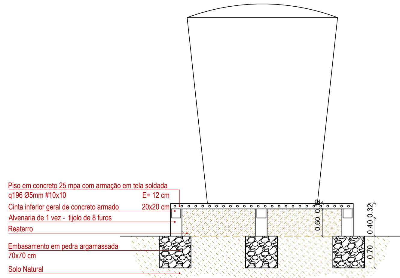
Corte AA – Base Reservatório Inferior escala 1/50
