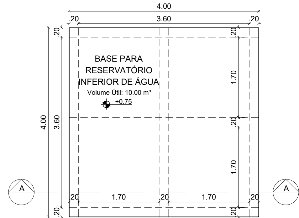
Planta Baixa – Base Reservatório Inferior escala 1/50
