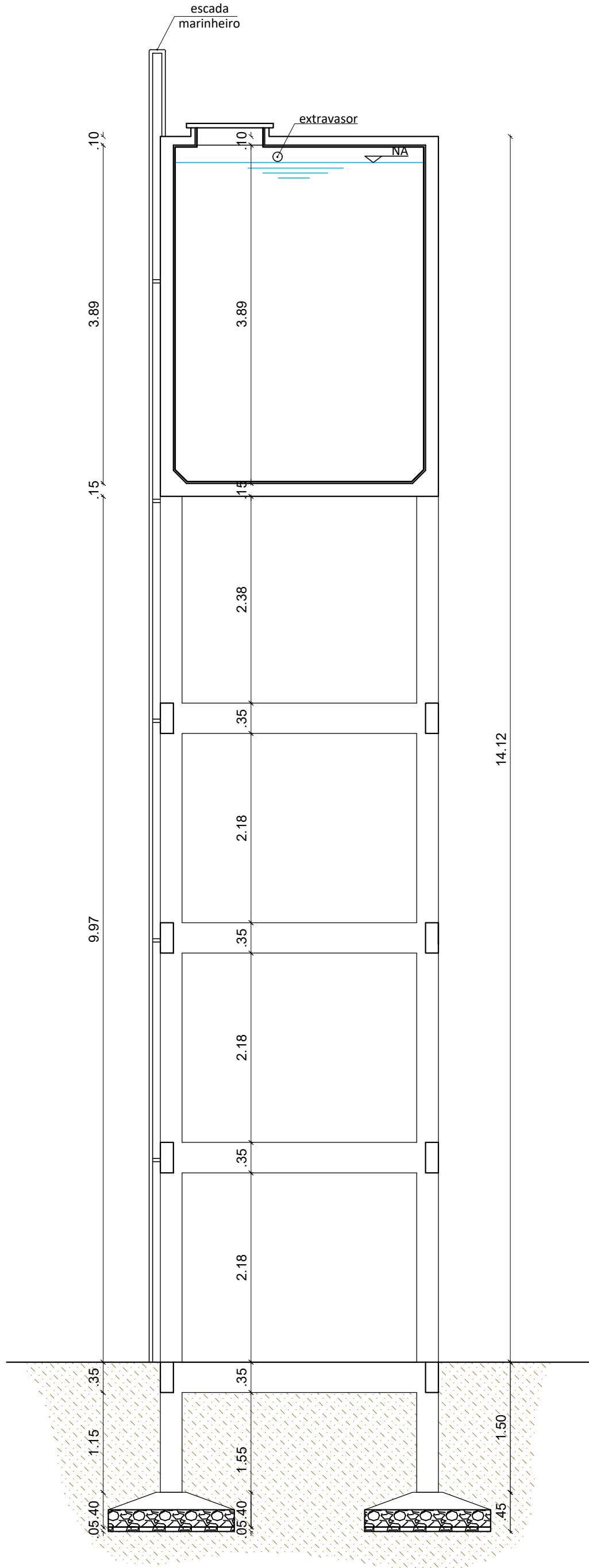
Corte AA – Reservatório Superior escala 1/50
