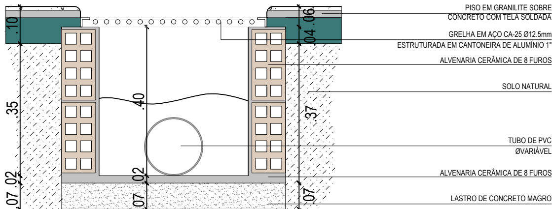
Detalhe – Grelha de drenagem escala 1/10
