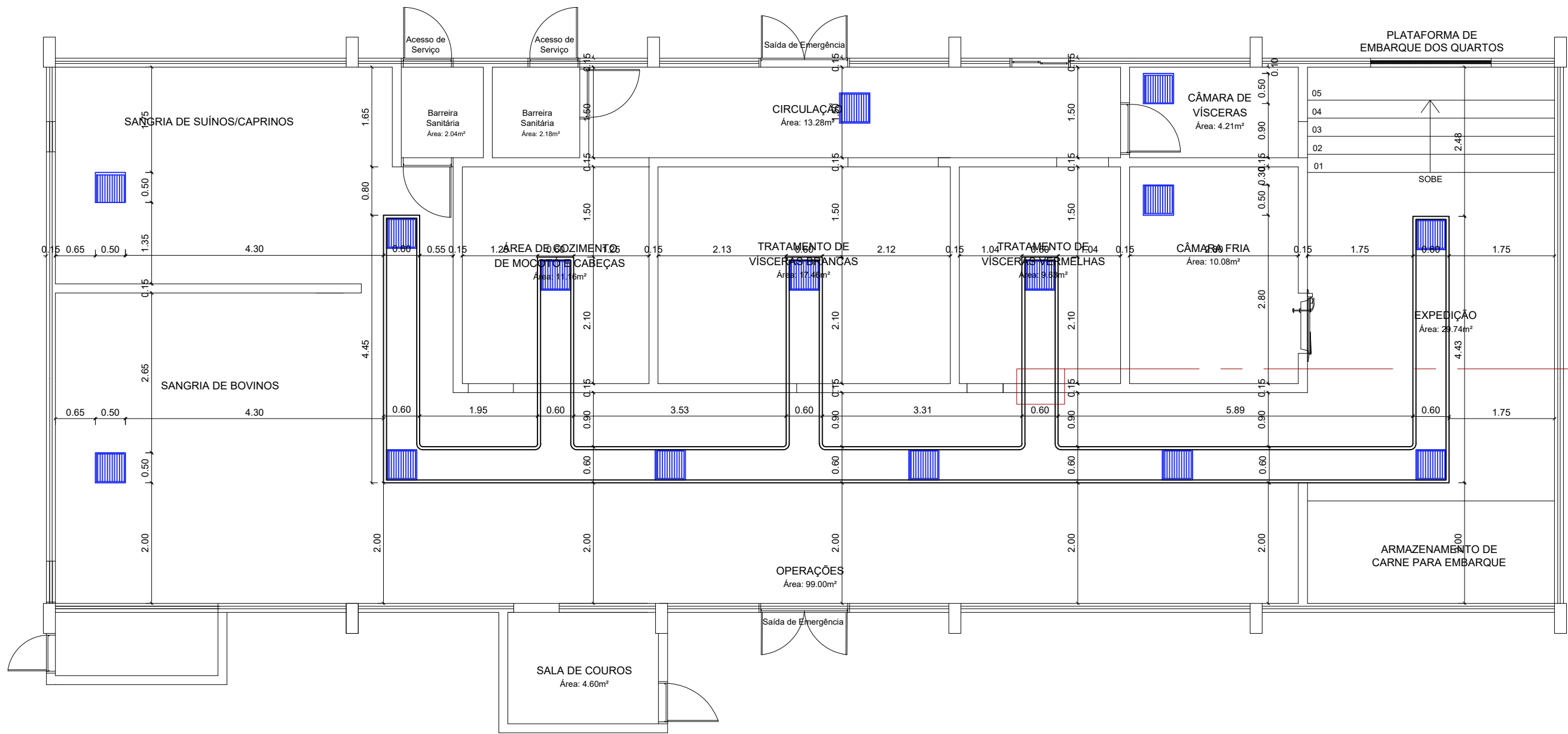
Planta Baixa Canaletas – Galpão escala 1/75
