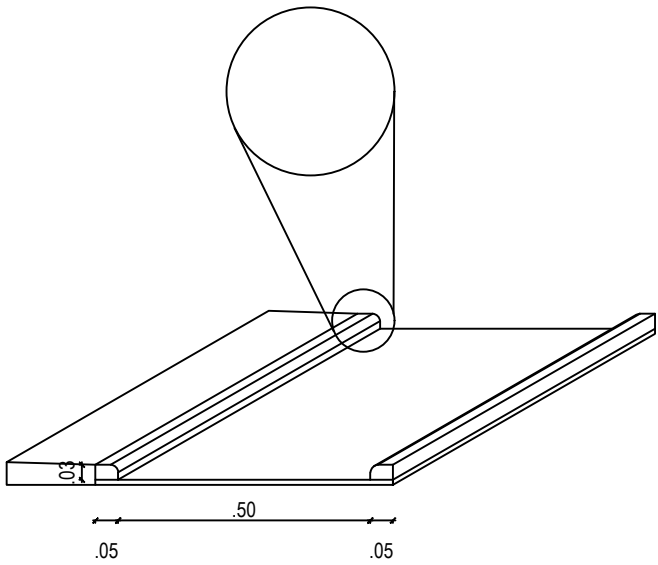
Detalhe – Canaleta escala 1/10
