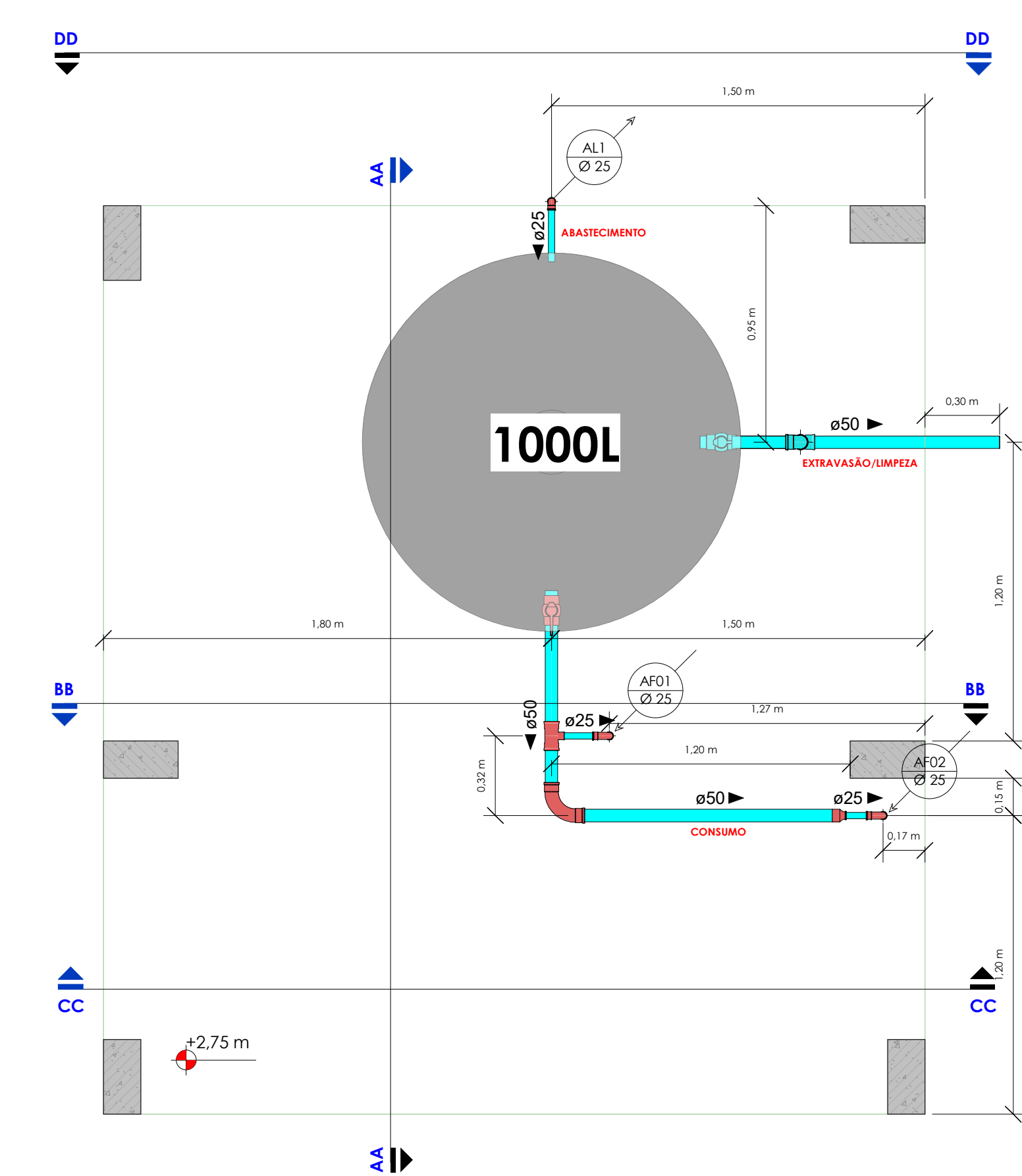
PLANTA BAIXA_COBERTA - CAIXA D'ÁGUA - ESC 1/20
