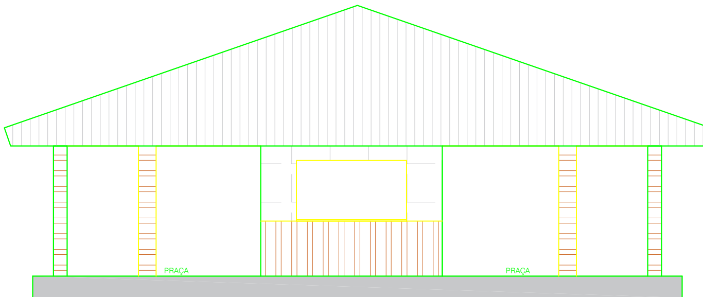
FACHADA NORTE QUIOSQUE ESCALA: 1/50
