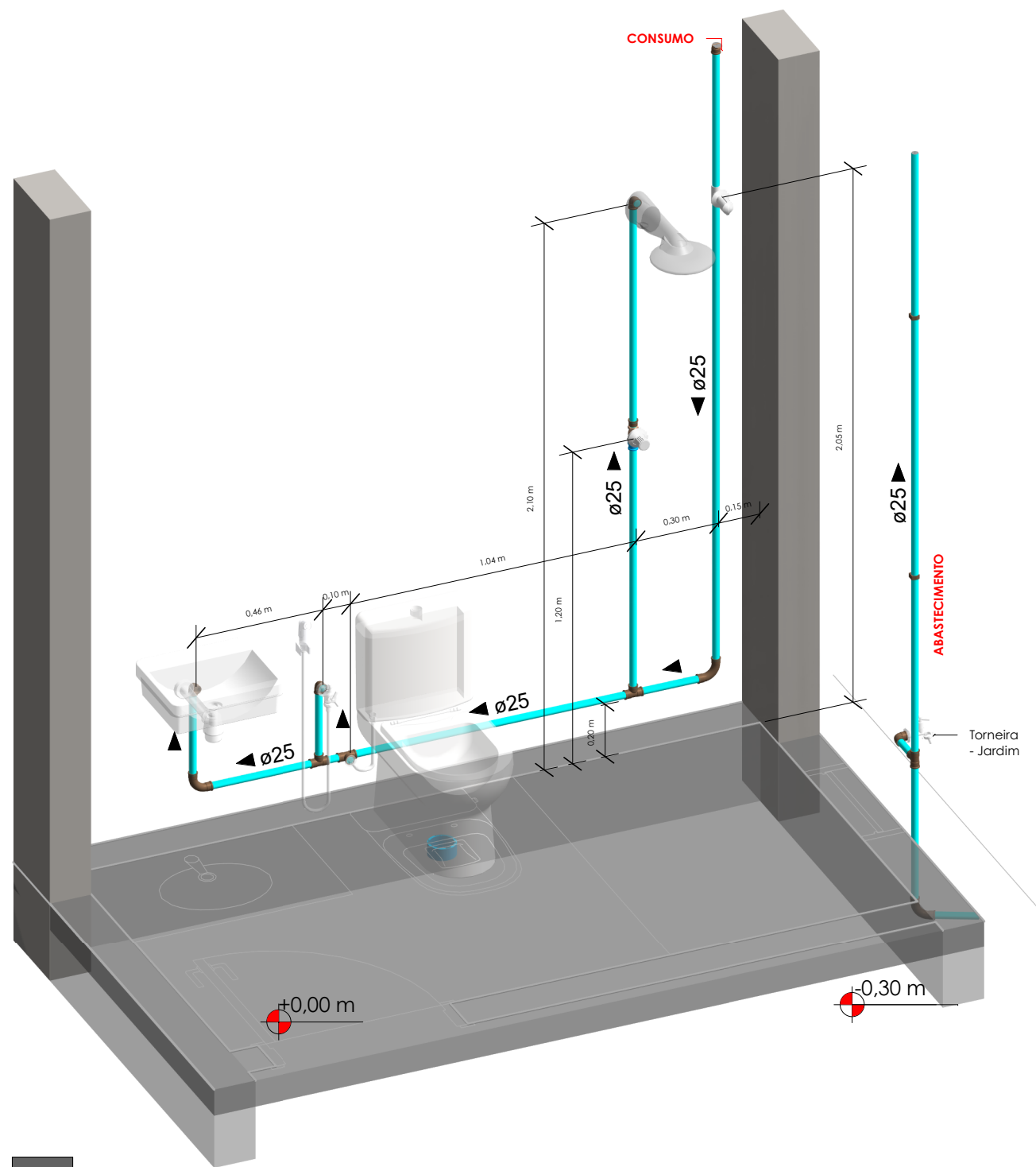
ISOMÉTRICA 01 - BWC GUARITA - ESC 1/20
