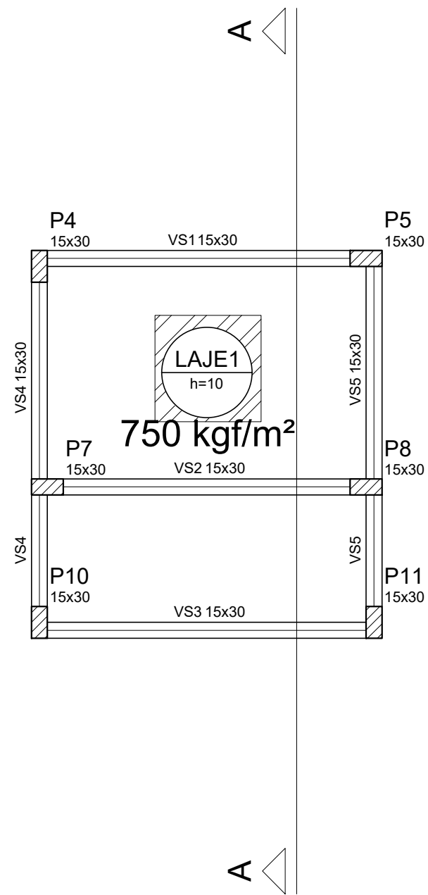
Forma do pavimento +270 escala 1:50
