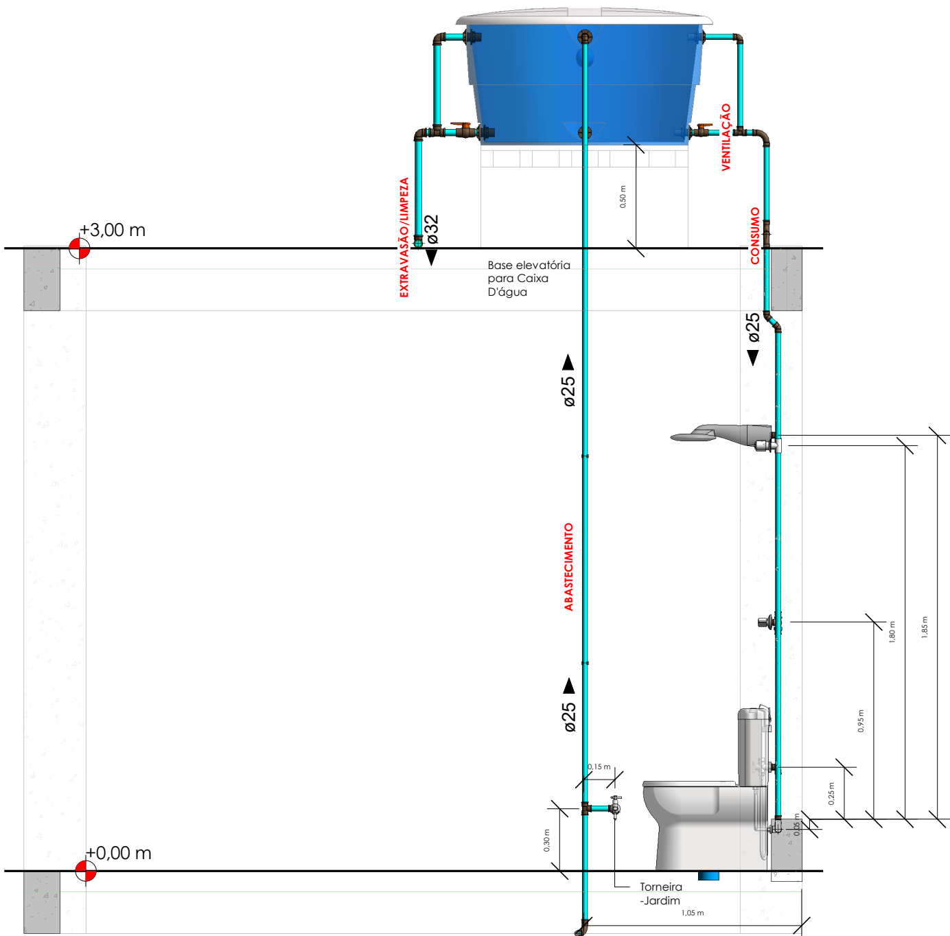
CORTE AA ESC 1/25
