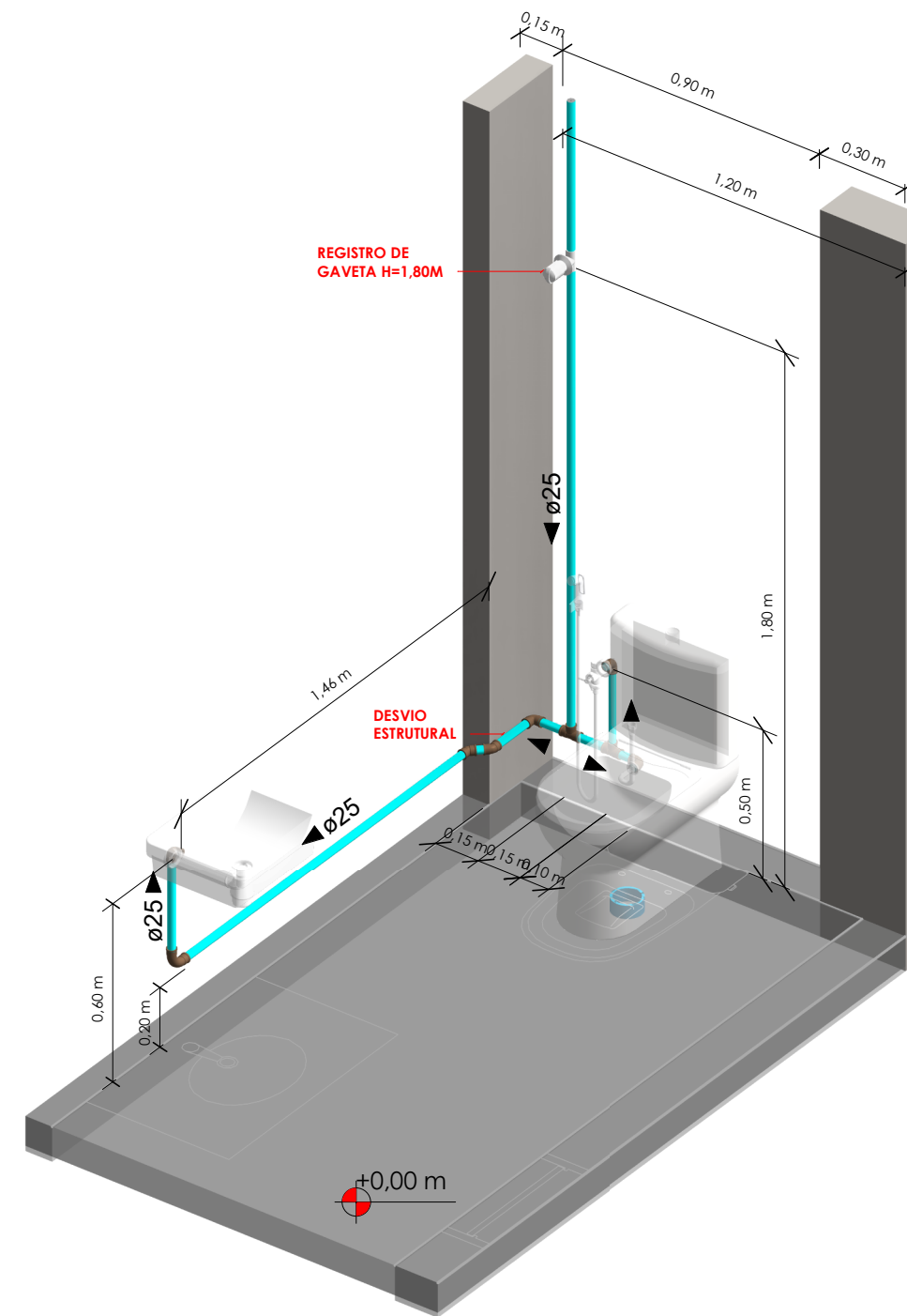
ISOMÉTRICA 01 - LAVABO - ESC 1/20
