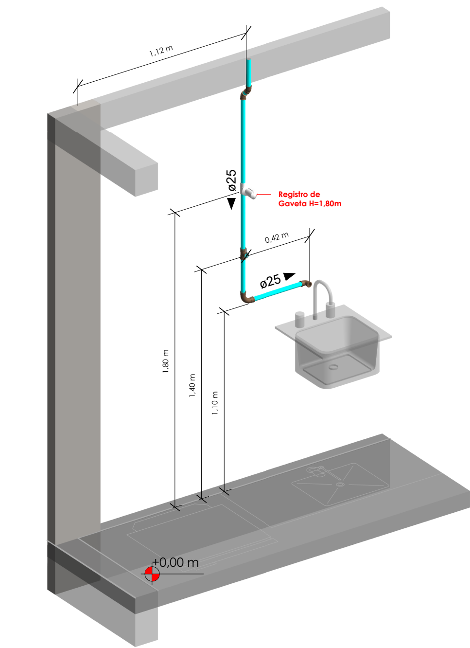
ISOMÉTRICA 02 - COZINHA - ESC 1/20
