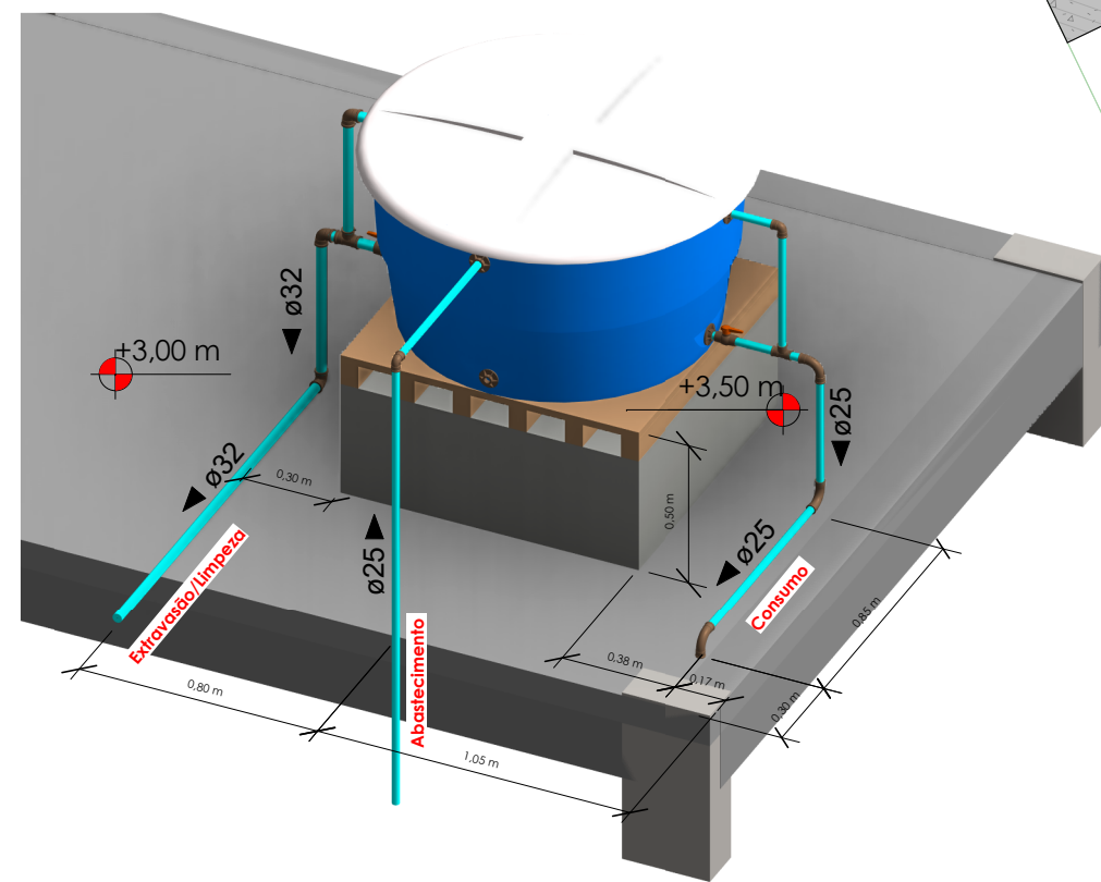
ISOMÉTRICA 02 - CAIXA_D'ÁGUA - ESC 1/25
