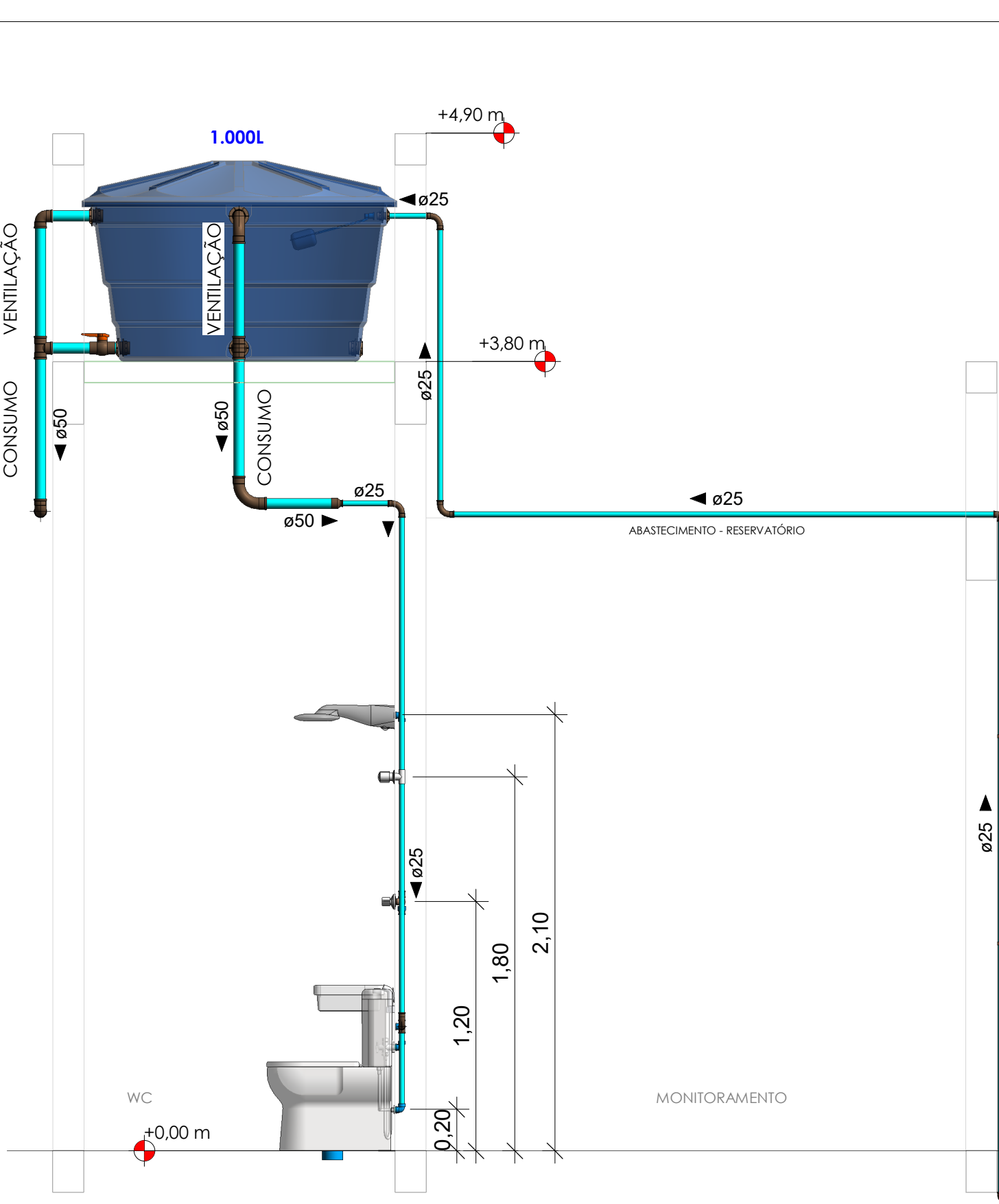
CORTE BB ESC 1/25
