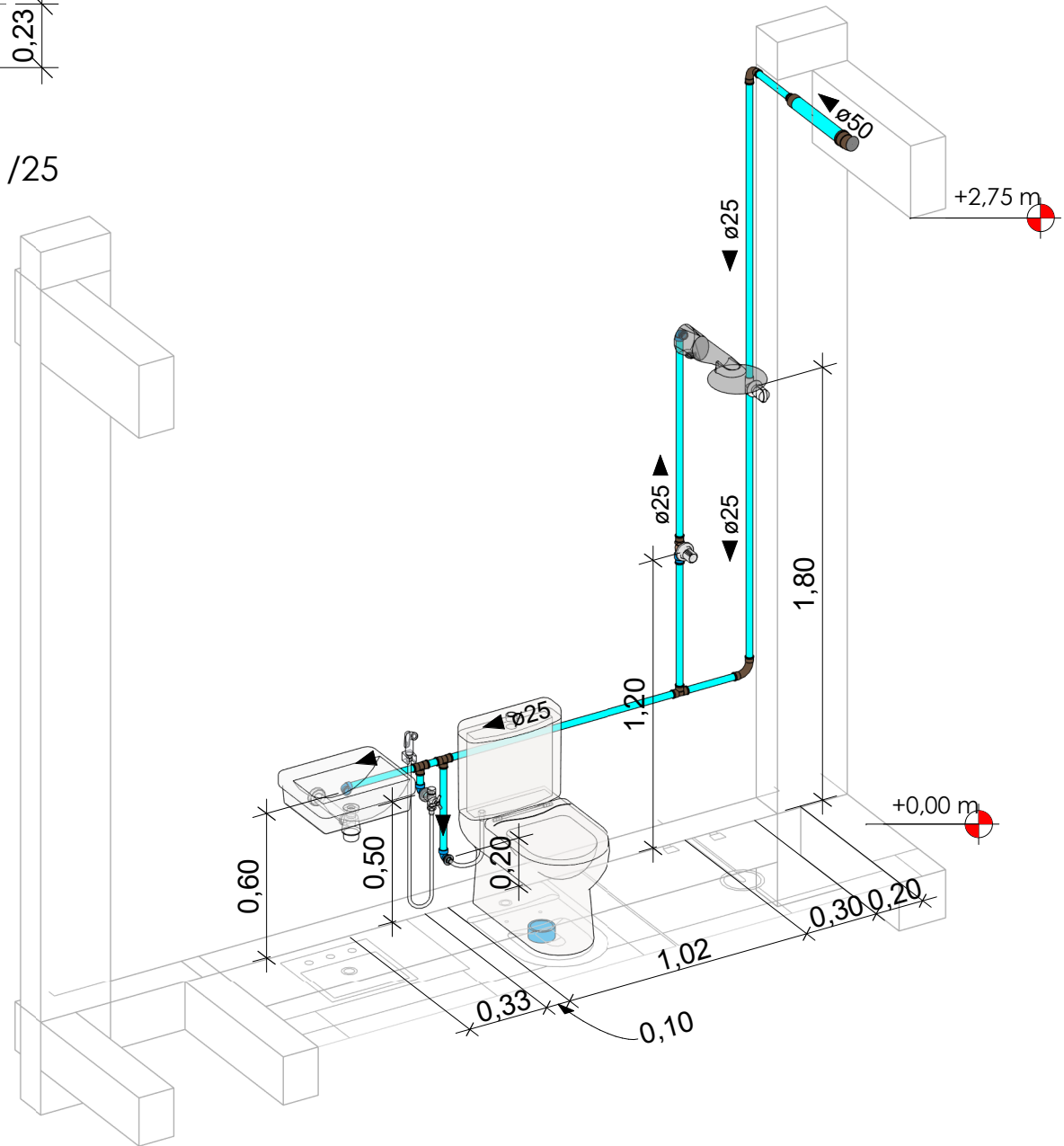
ISOMÉTRICA 01 - WC 1 - ESC 1/25
