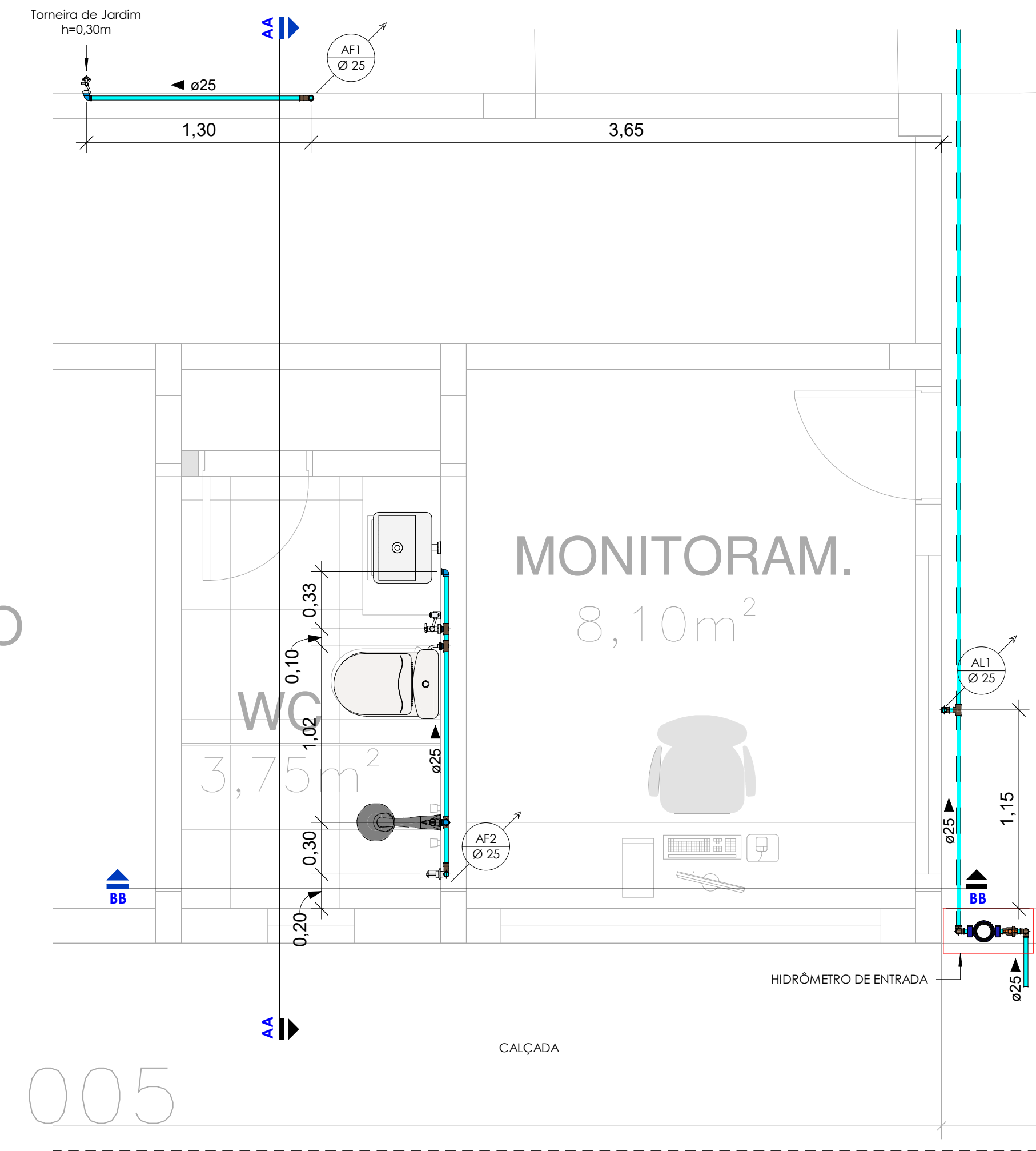
PLANTA BAIXA_ REFORMA_GARAGEM_TÉRREO_DORMITÓRIO_WC_MONITORAMENTO - ESC 1/25
