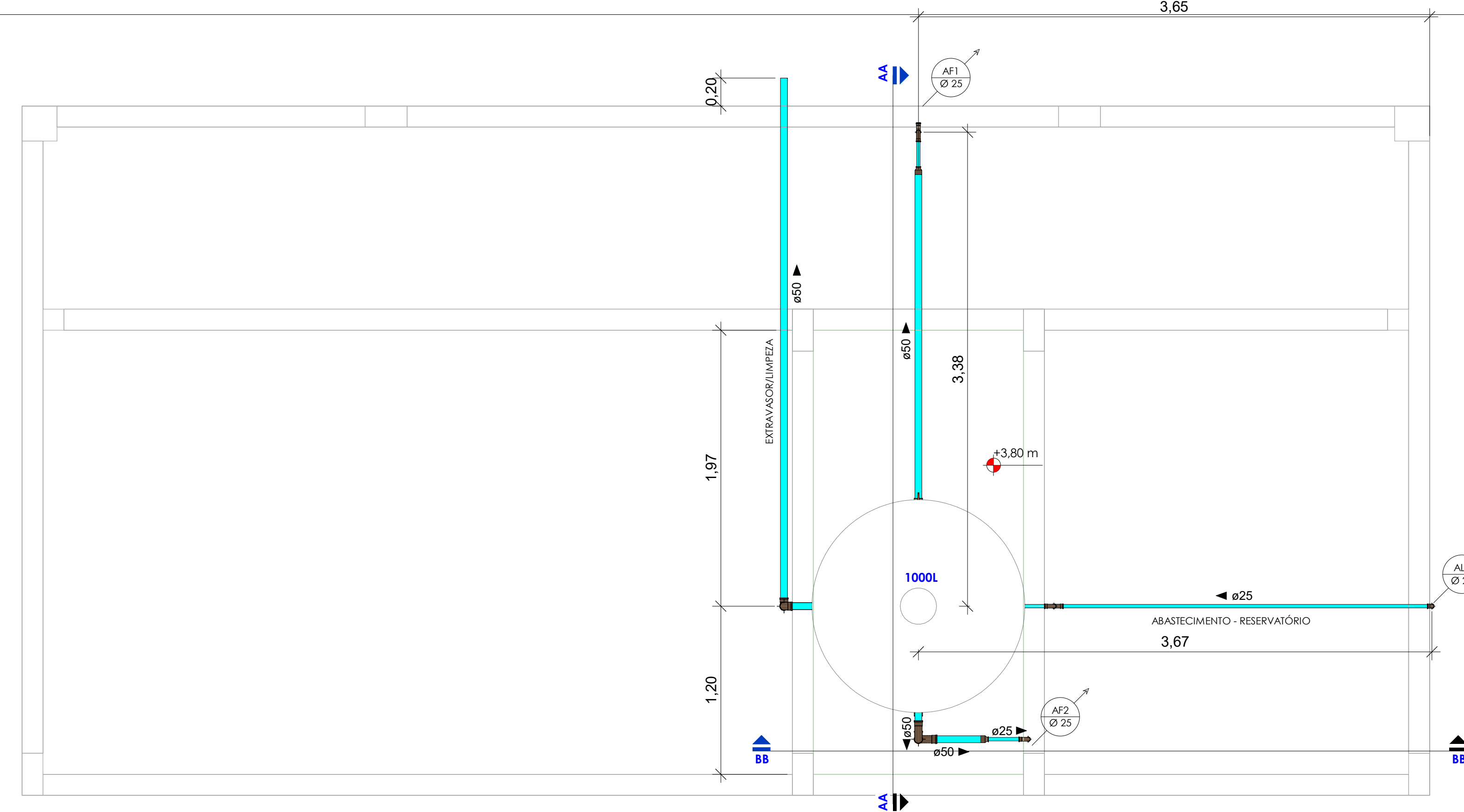
PLANTA BAIXA_ COBERTA - CAIXA_ D'ÁGUA_01 - ESC 1/25
