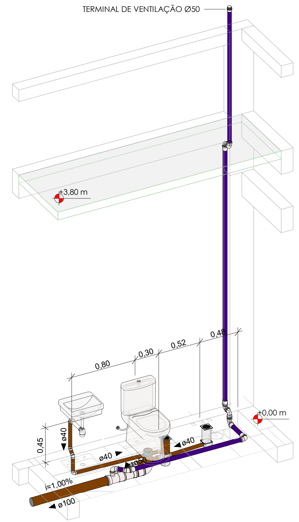
ISOMÉTRICA 02 - WC_MONITORAMENTO - ESC _____ 1/25
