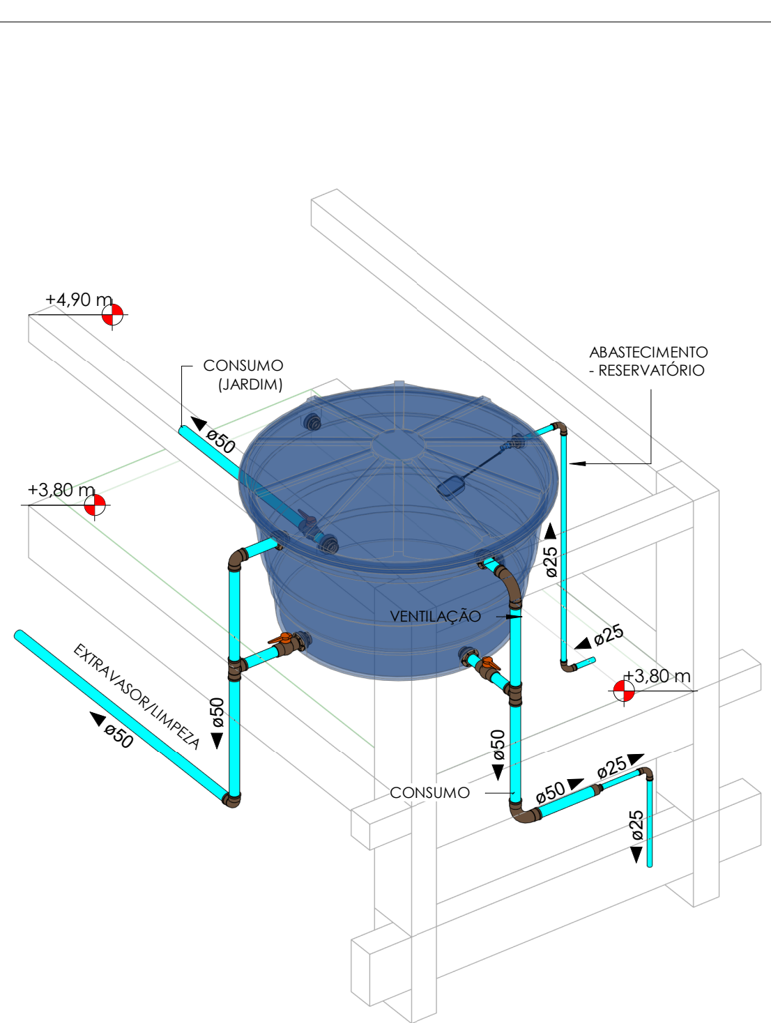
ISOMÉTRICA 02 - WC 2 - ESC 1/25
