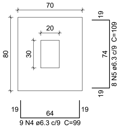
S1=S14 PLANTA ESC 1:25
