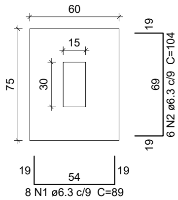
S1=S14 PLANTA ESC 1:25
