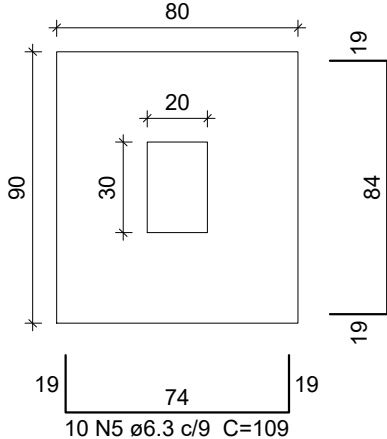
S6=S9 PLANTA ESC 1:25
