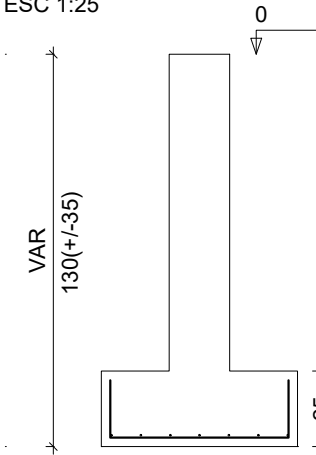
CORTE ESC 1:25
