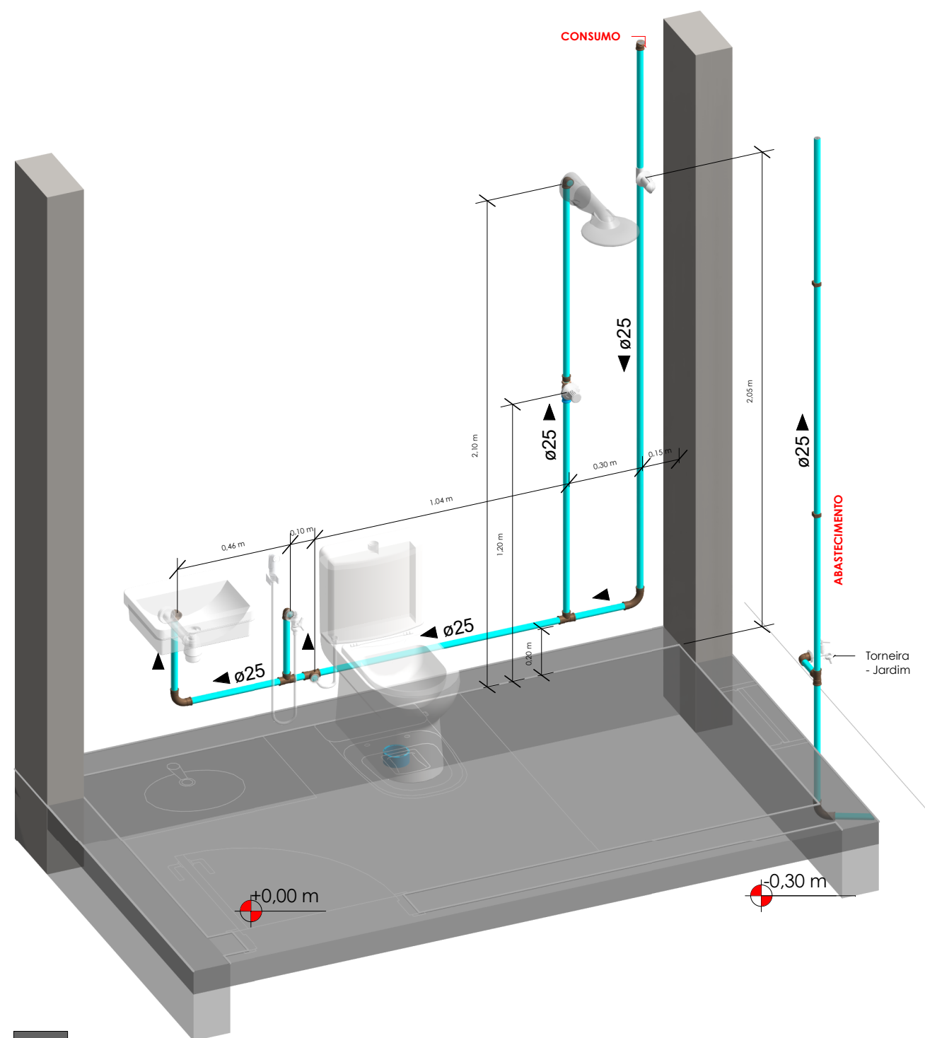
ISOMÉTRICA 01 - BWC GUARITA - ESC
