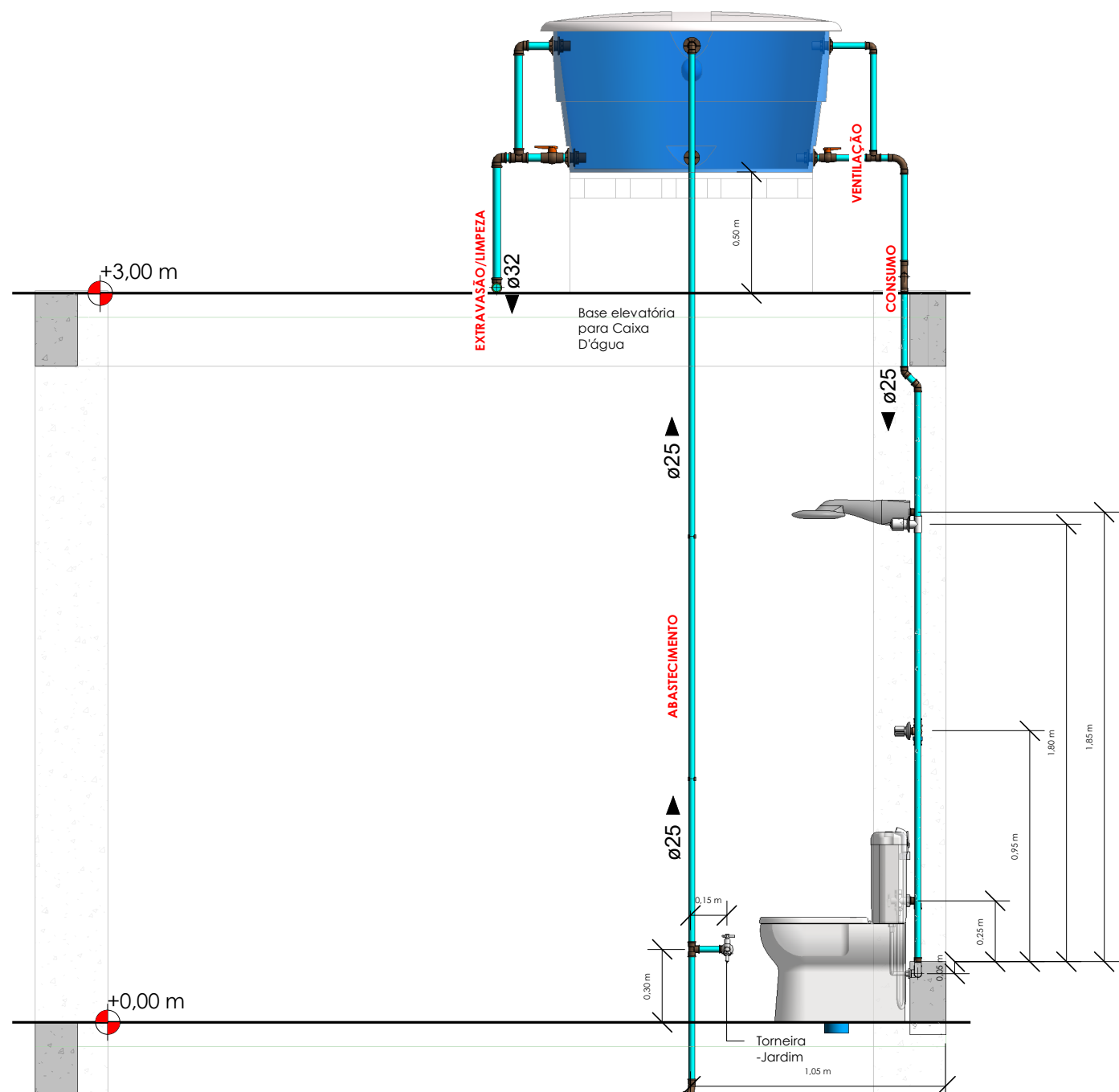
CORTE AA
