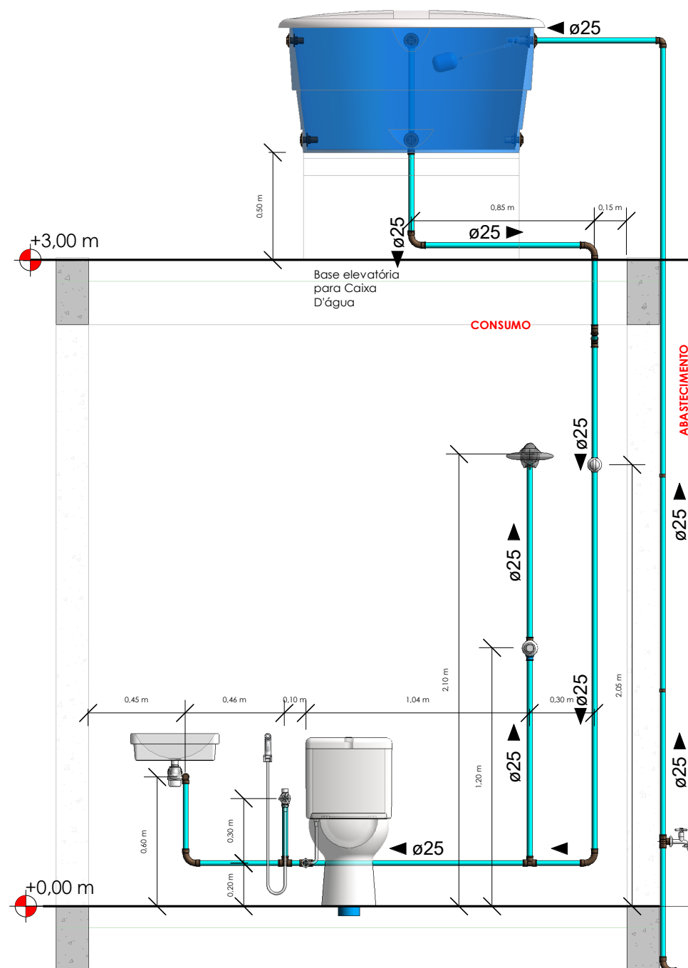
CORTE BB
