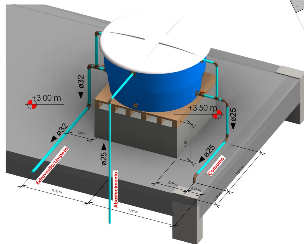
ISOMÉTRICA 02 - CAIXA_D'ÁGUA - ESC
