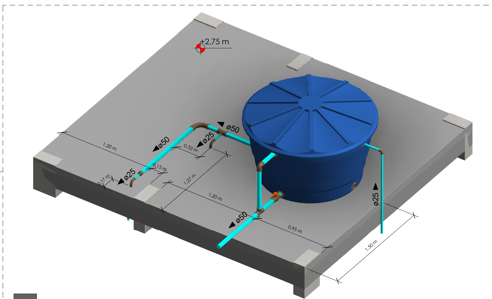
ISOMÉTRICA 03 - CAIXA D'ÁGUA - ESC 1/25
