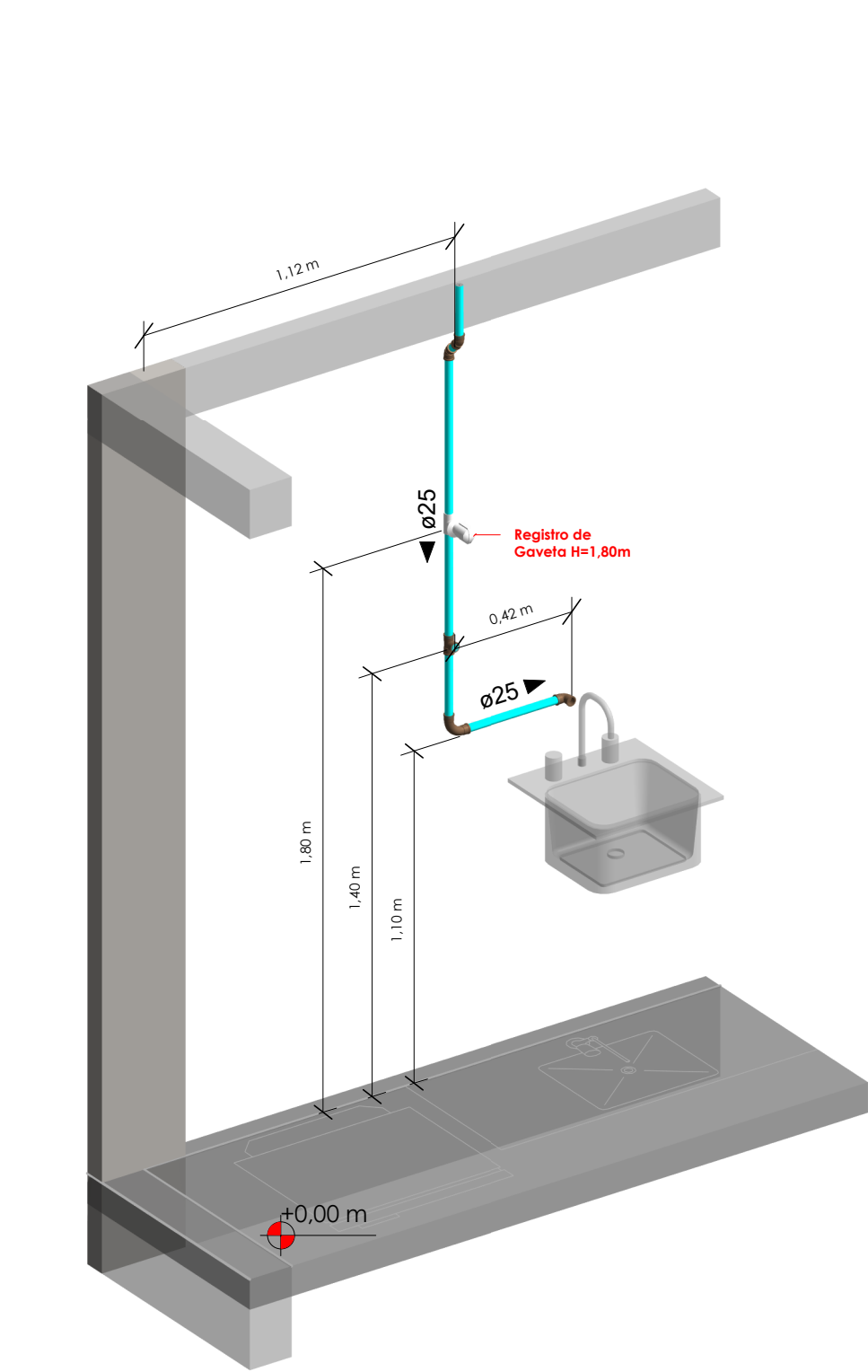
ISOMÉTRICA 02 - COZINHA - ESC 1/20
