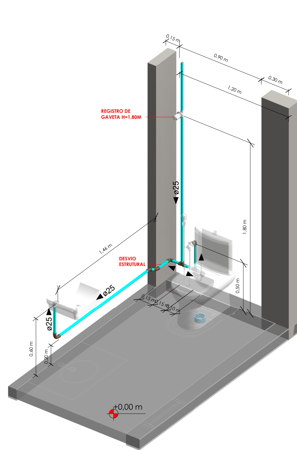
ISOMÉTRICA 01 - LAVABO - ESC 1/20
