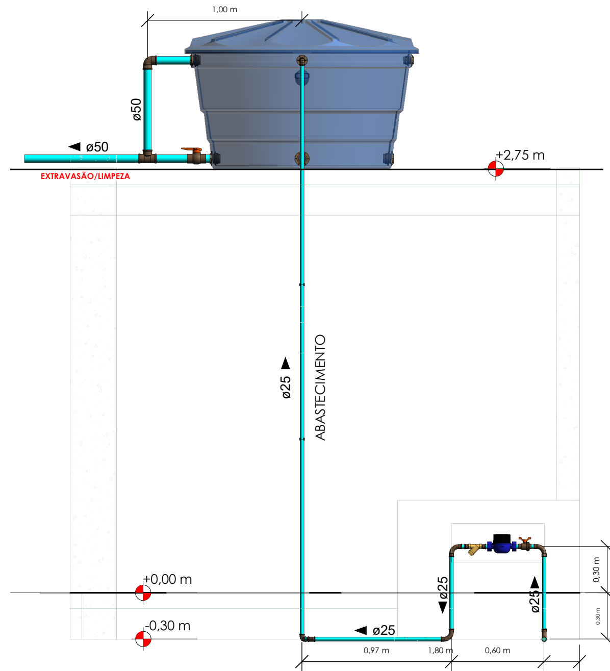
CORTE DD ESC 1/25
