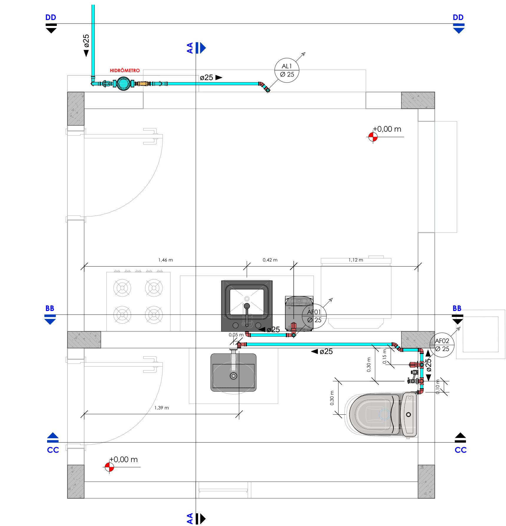
PLANTA BAIXA_TÉRREO QUIOSQUE_PRAÇA_NOVA_COREMAS - ESC 1/20
