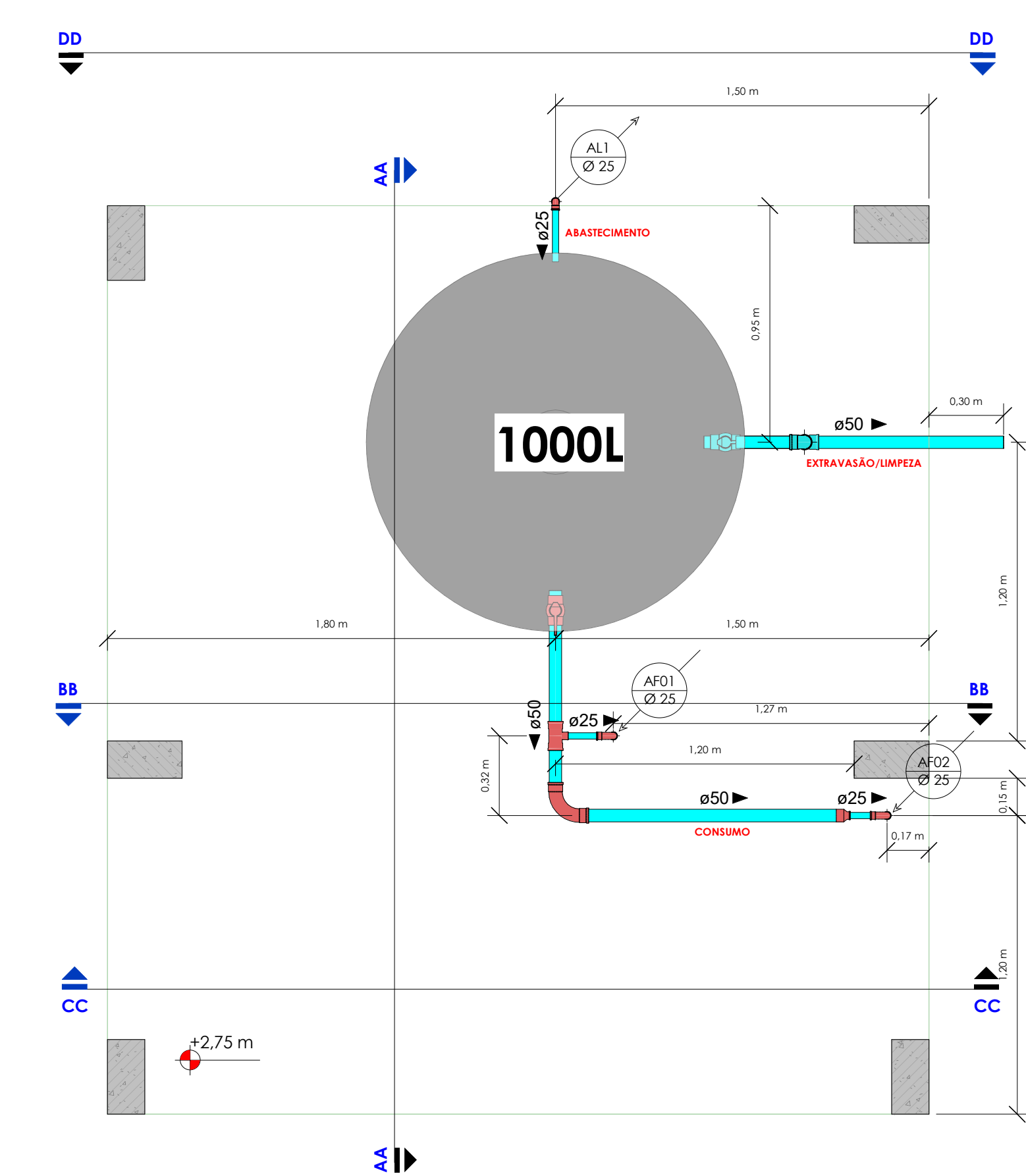
PLANTA BAIXA_COBERTA - CAIXA_D'ÁGUA - ESC 1/20
