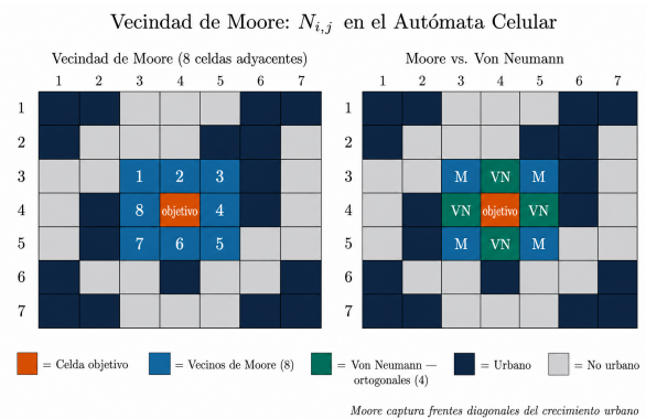
Figura 5.5: Vecindad de Moore (8 celdas) frente a Von Neumann (4 ortogonales). Moore captura frentes diagonales de crecimiento.
