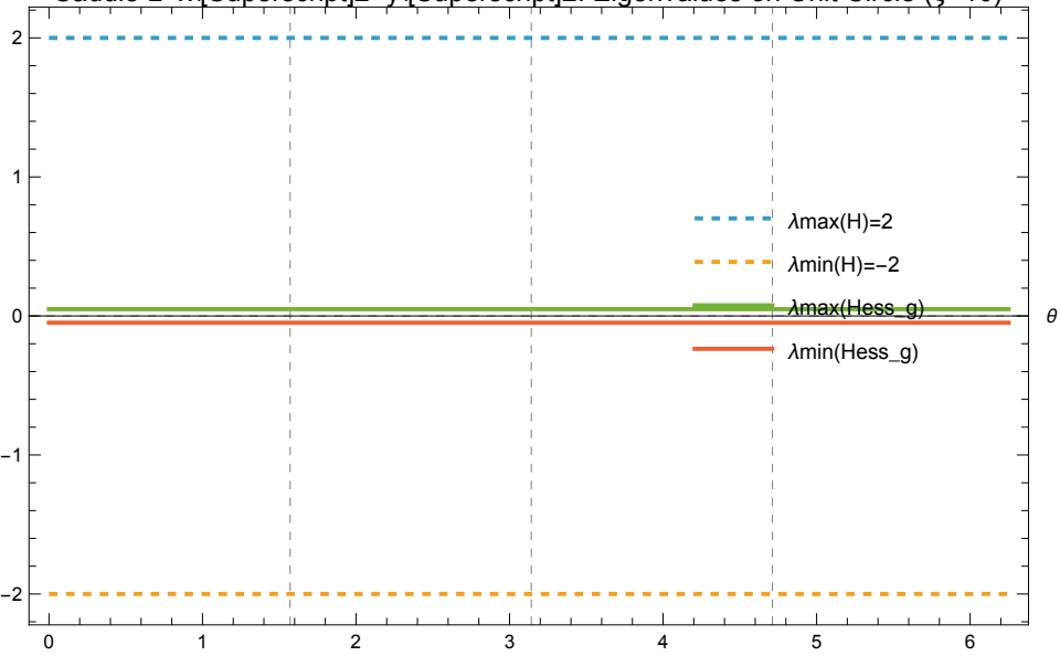
Saddle L=x^{[2]}-y^{[2]} : Eigenvalues on Unit Circle ( \xi=10 )
