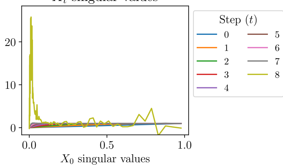
X_t singular values
