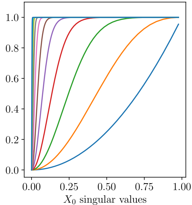
R_t eigenvalues
