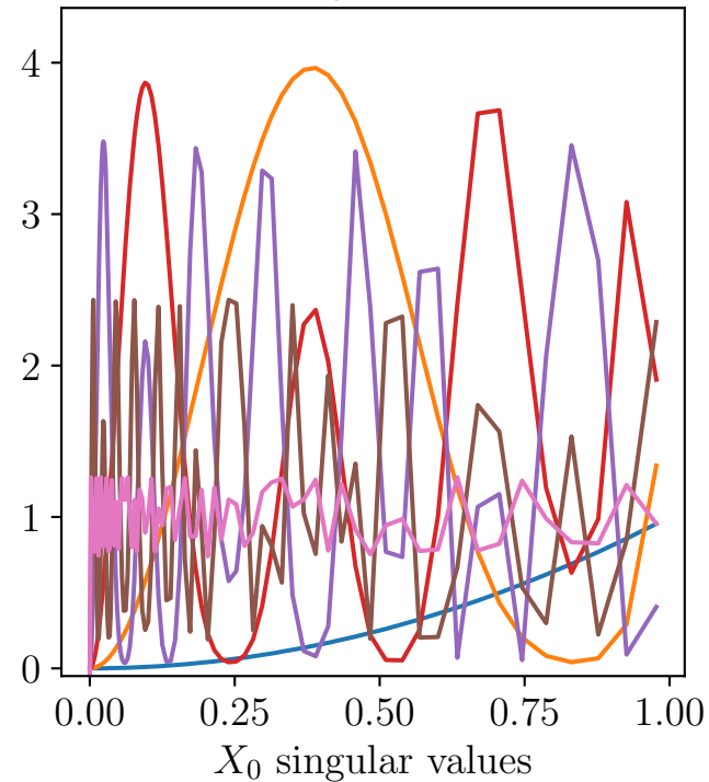
R_t eigenvalues
