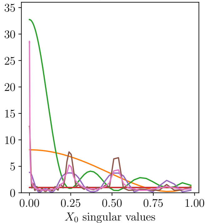
Q_t eigenvalues
