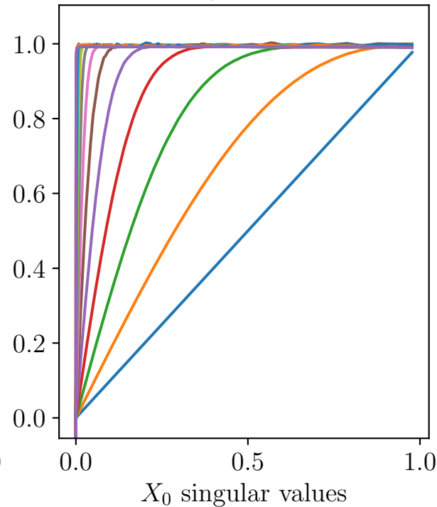
X_t singular values
