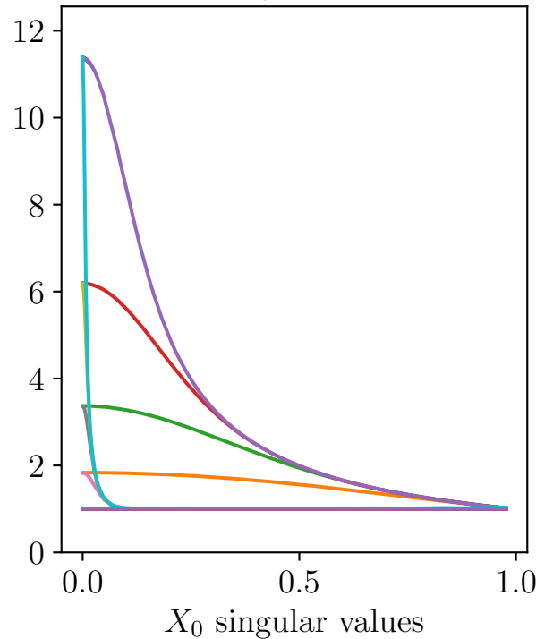
Q_t eigenvalues
