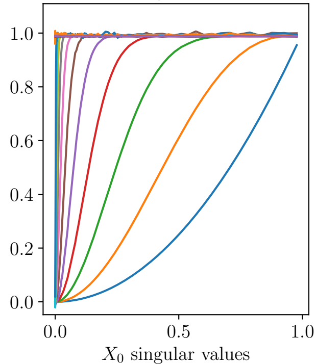
R_t eigenvalues
