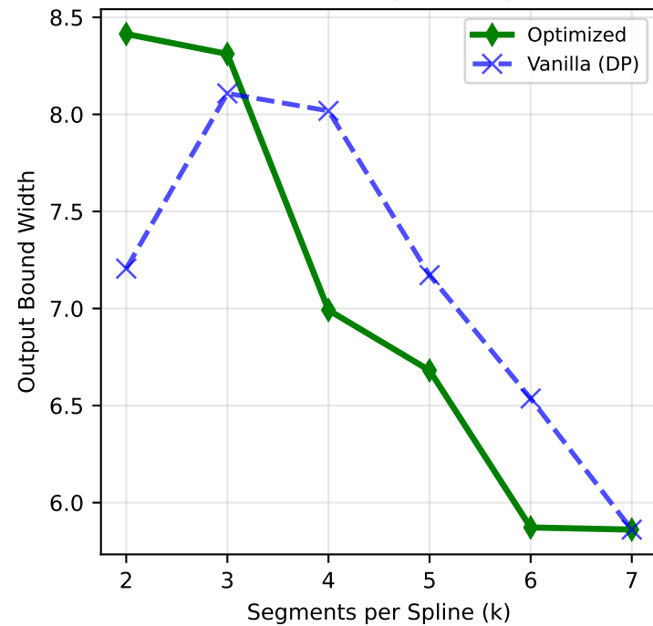
Small -- functionexp4 (260 params)
