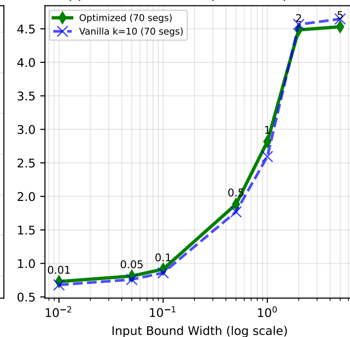
Appendix-2 -- funcellipeinc (70 params)
