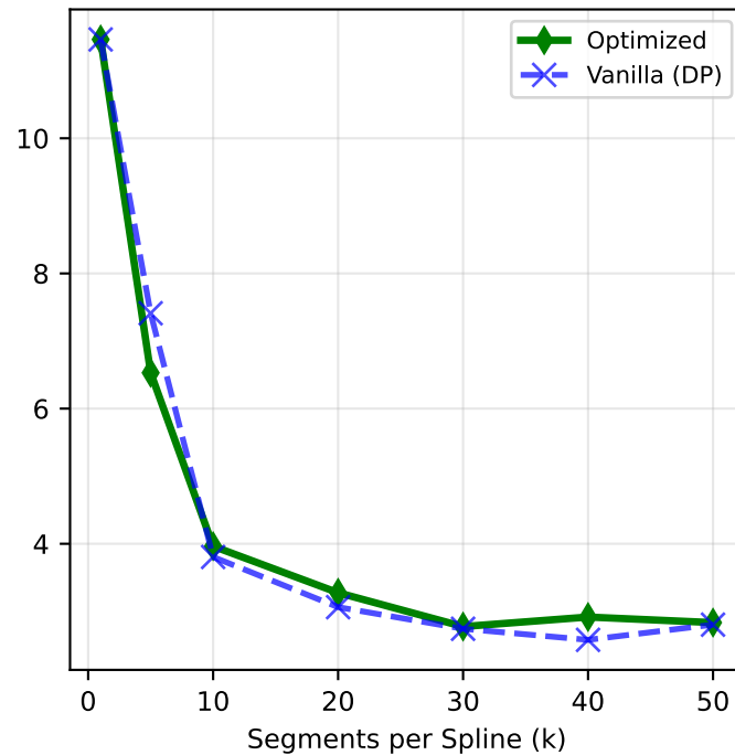
Medium -- functionexp4 (260 params)
