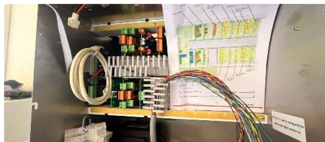
Coffret CAHORS ouvert avec plan de raccordement des cartes
