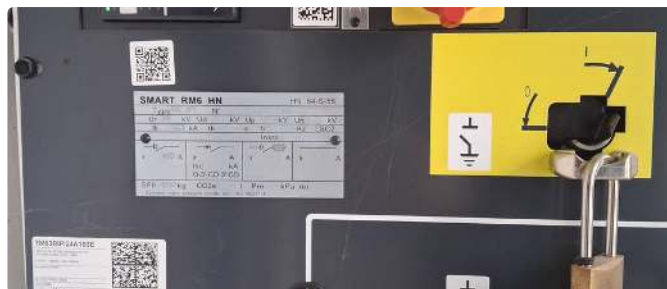
Cellule Smart RM6 HN — schéma unifilaire et interface OMT intégrée
