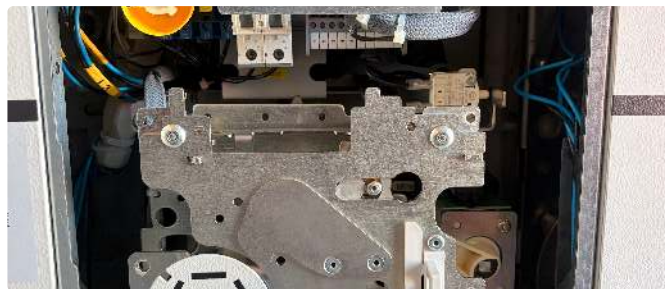
Tore WEGA ZERO et PPACS sur cellule ouverte — mesures Ir et Vr
