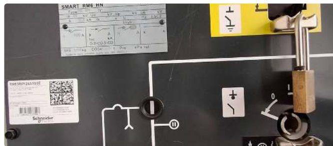
Cellule Smart RM6 HN — plaque signalétique et interface OMT intégrée
