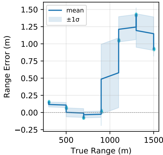
Range error vs true range
