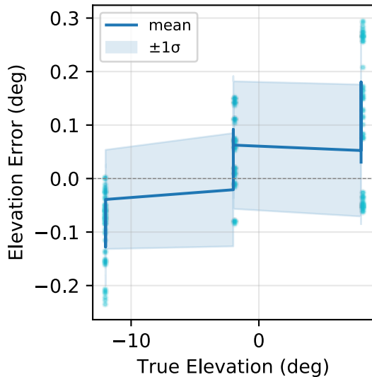
Elevation error vs true elevation
