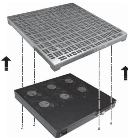
(图 3-d) 「辅助空调模块」锁附于高架地板下
