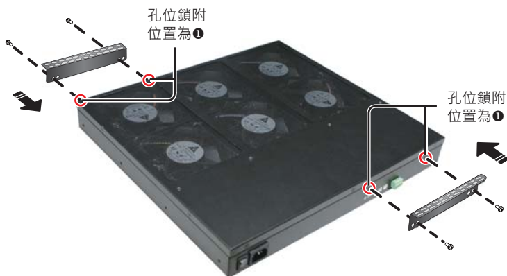
(圖 3-c)「輔助空調模組」支架鎖附圖
