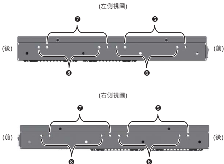
(圖 3-b)「輔助空調模組」孔位鎖附位置 (左 / 右側)
