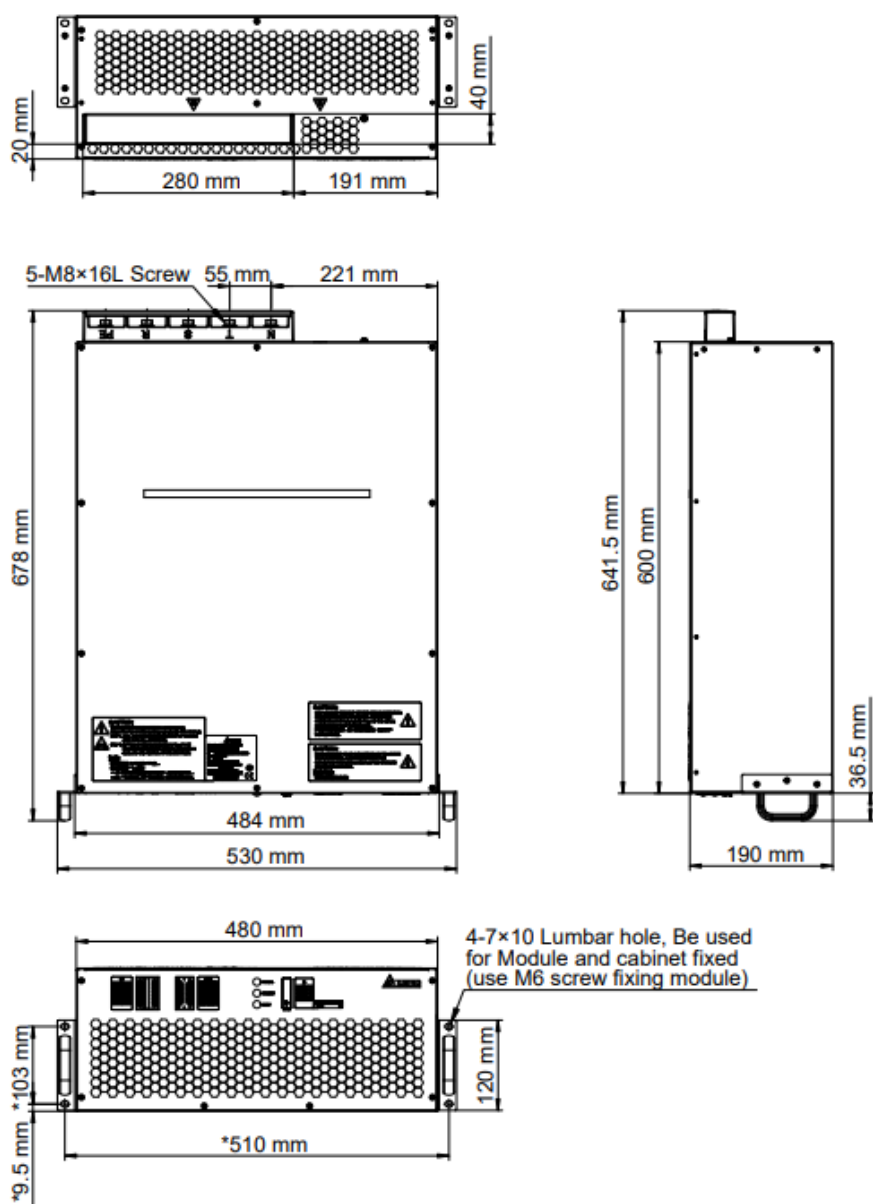
(Figure 3-10: SVG Module Dimensions_ 50kvar Models)
