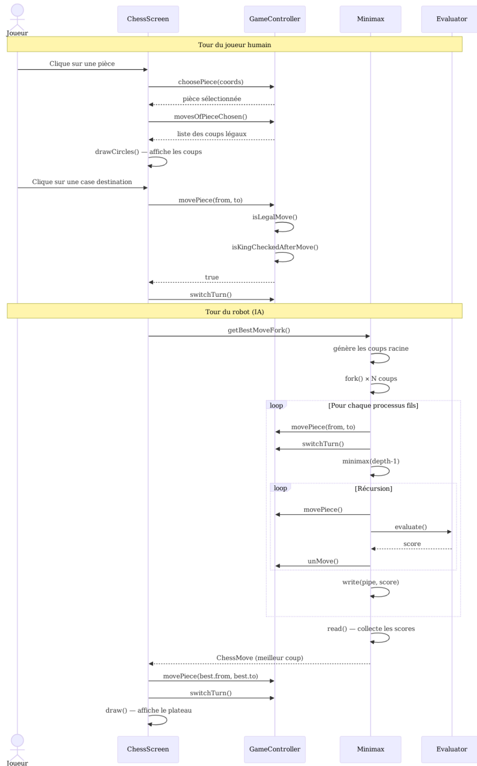
Figure 8: Diagramme de séquence UML
