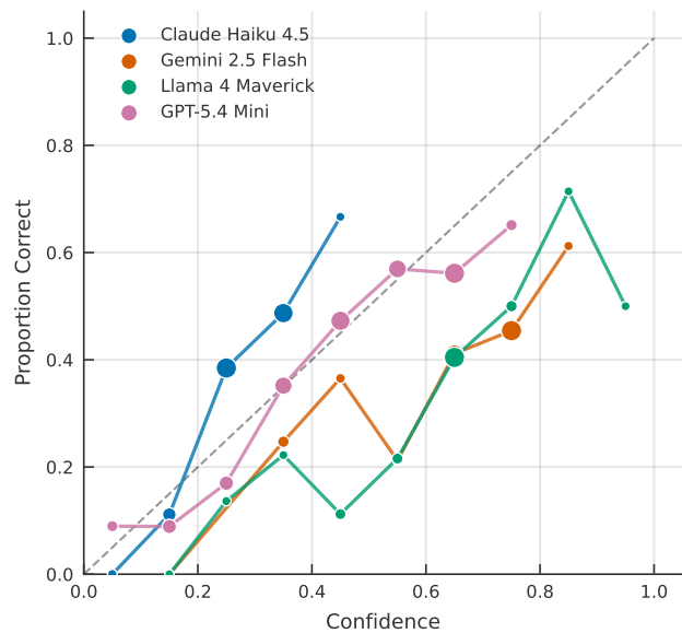
WGD
