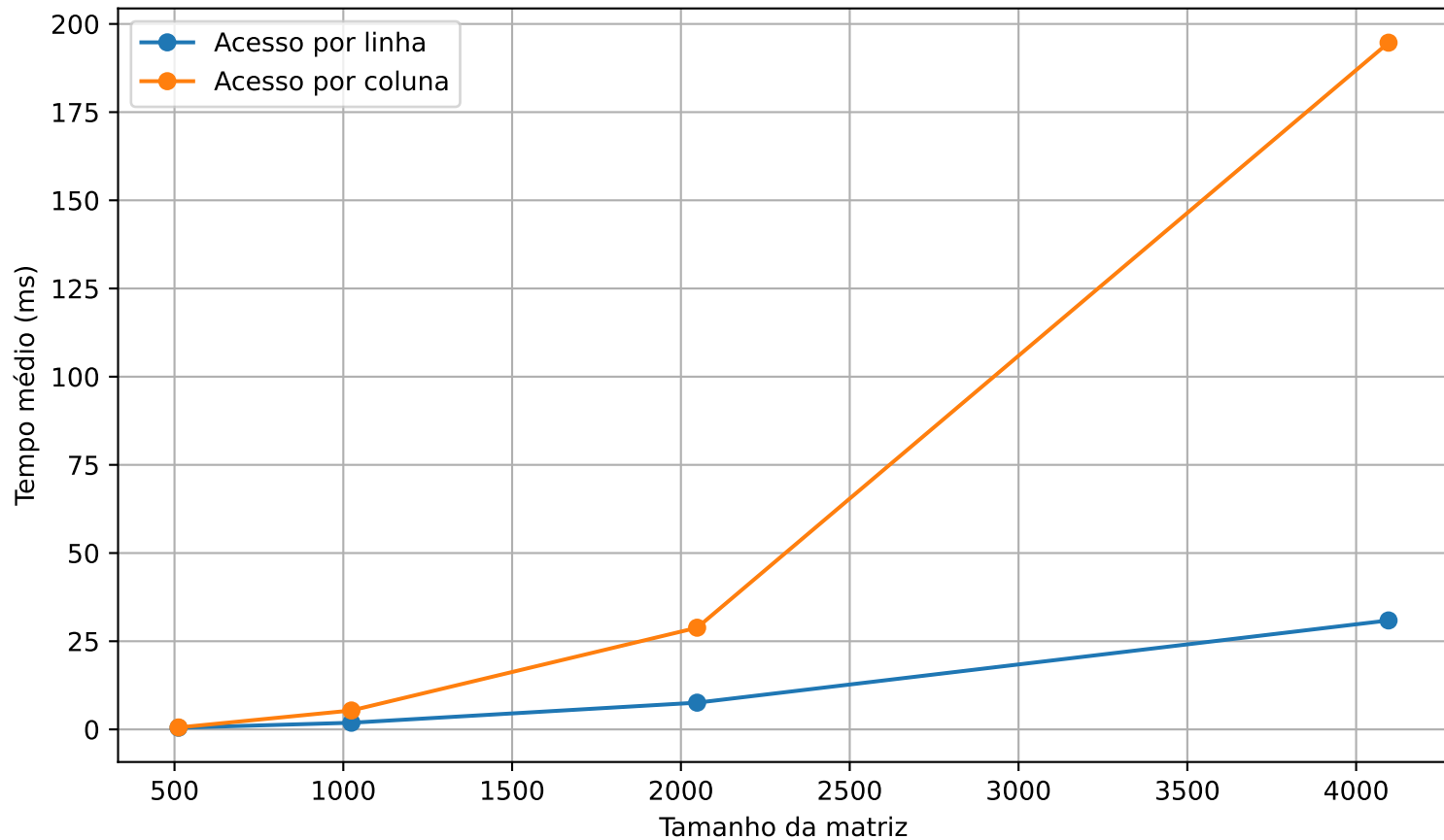
Tempo médio por padrão de acesso - O0
