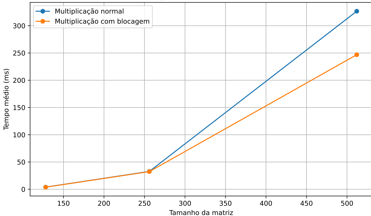
Multiplicação de matrizes - O0
