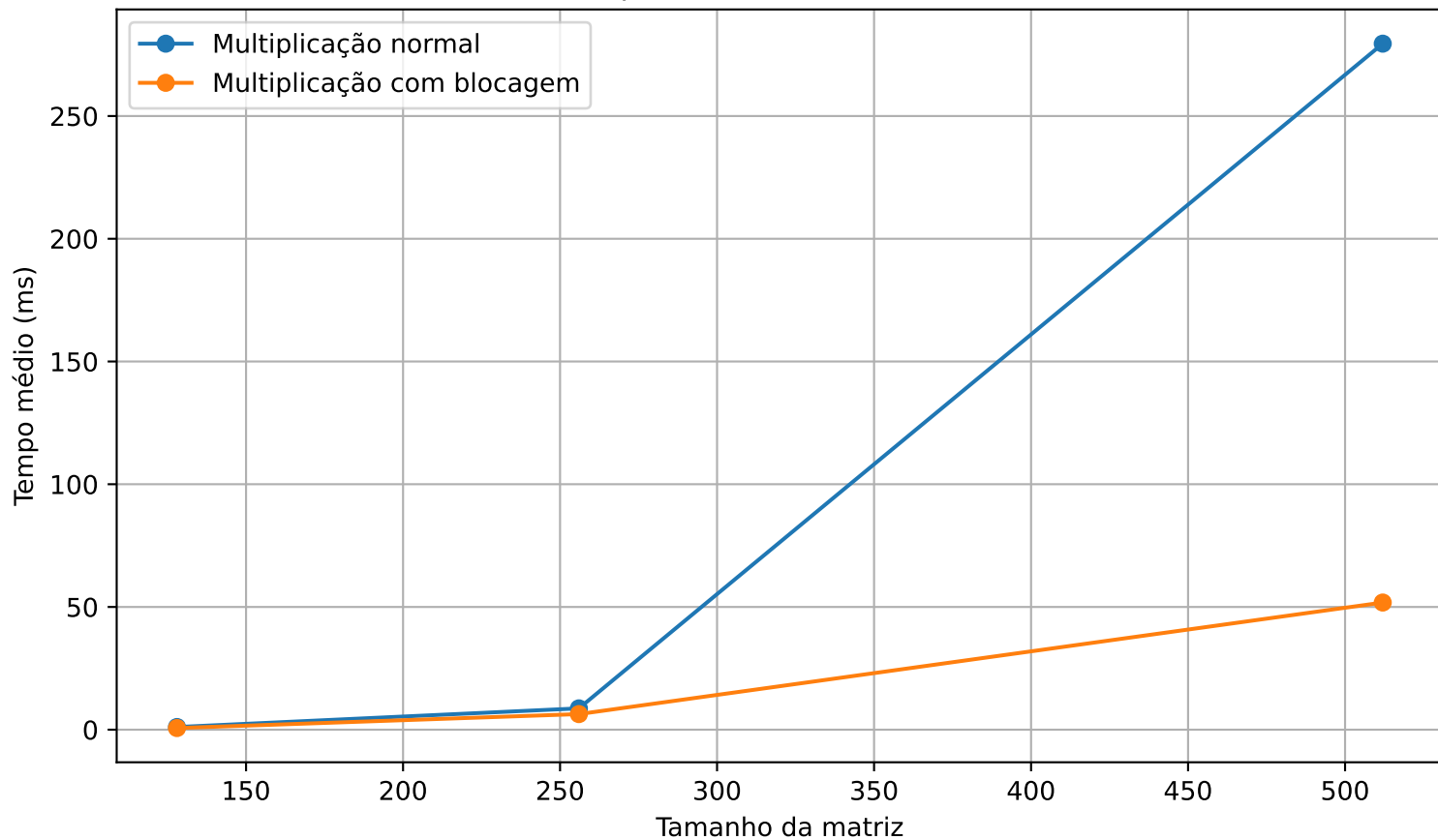
Multiplicação de matrizes - O2
