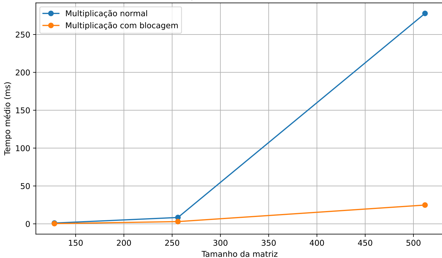
Multiplicação de matrizes - O3
