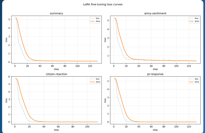
4개 LoRA 태스크 학습 곡선
