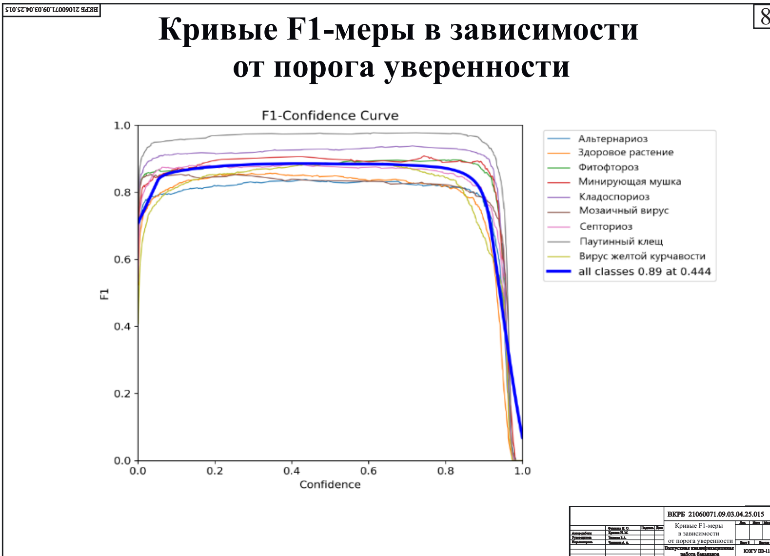
Рисунок А.8 – Кривые F1-меры в зависимости от порога уверенности
