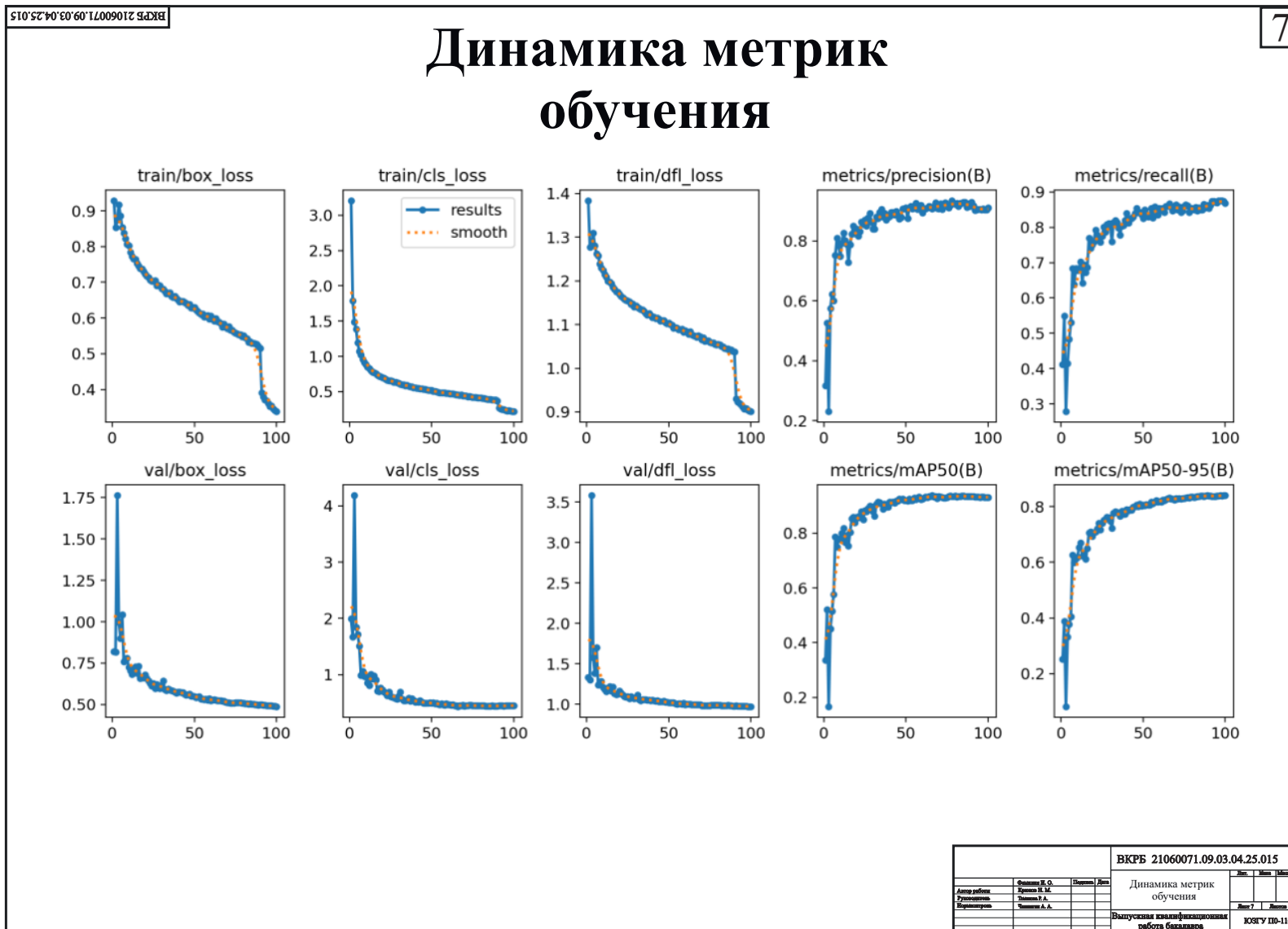
Рисунок А.7 – Динамика метрик обучения
