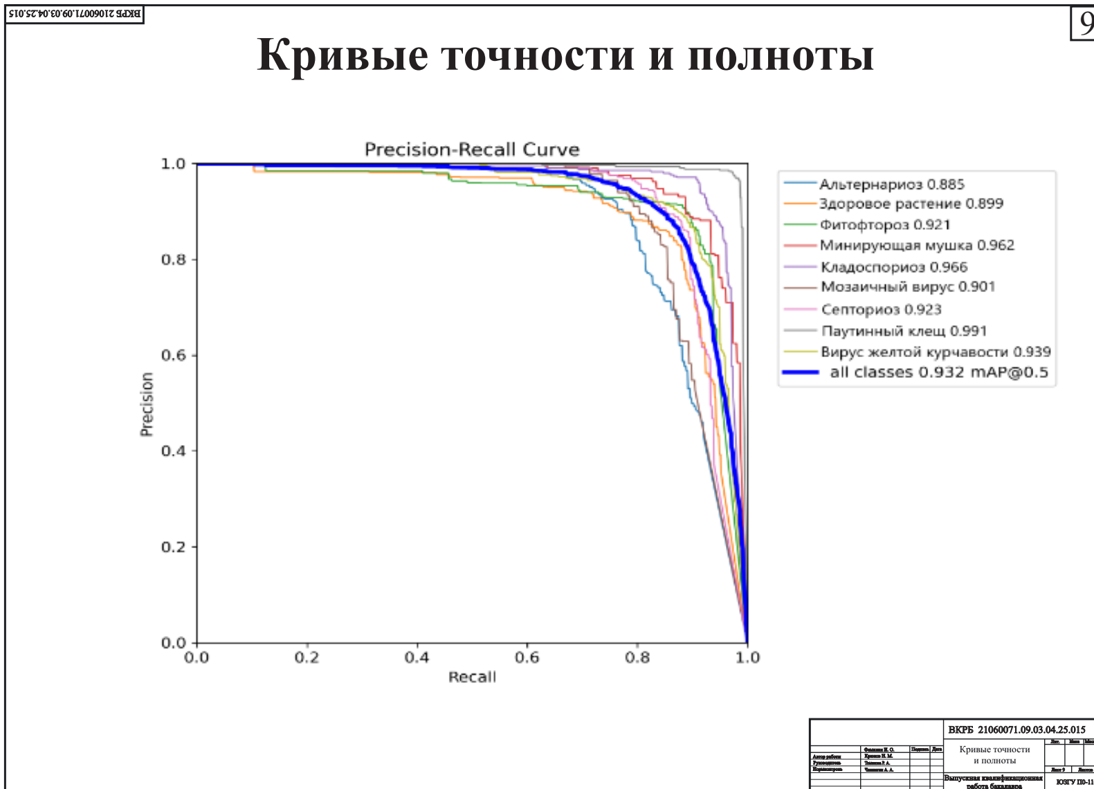
Рисунок А.9 – Кривые точности и полноты
