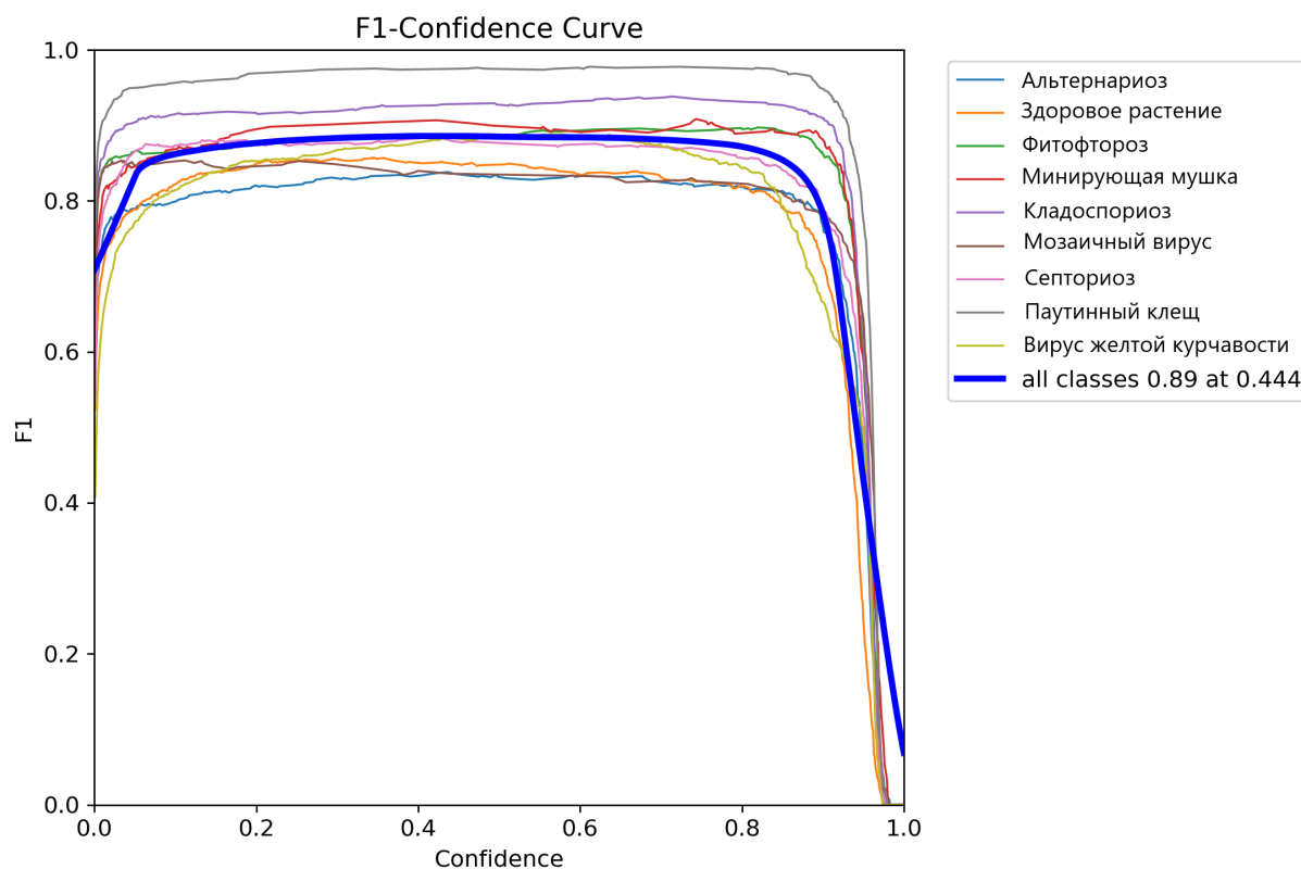
Рисунок 4.2 – Кривые F1-меры в зависимости от порога уверенности.
