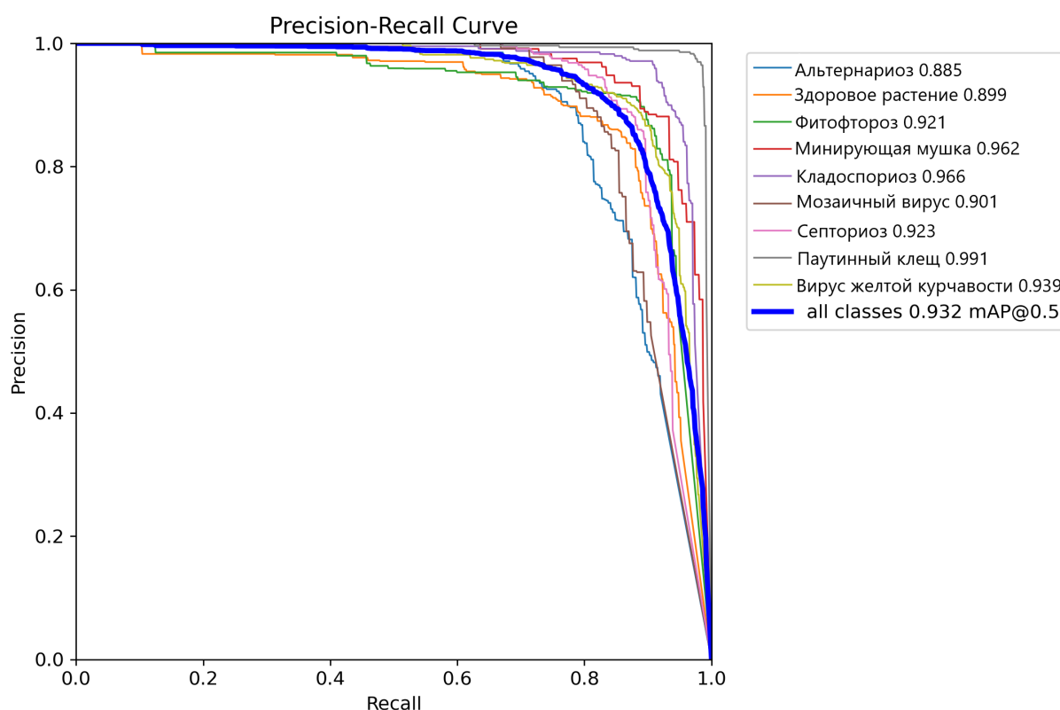
Рисунок 4.3 – Кривые точности и полноты
