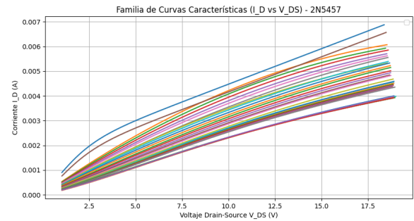
Fig. 14: Familia completa de curvas características de drenador reales extraídas para el JFET bajo estudio.
