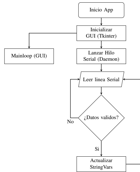
Fig. 9. Diagrama de flujo de la arquitectura multihilo de la aplicación en Python ( visual.py ).
