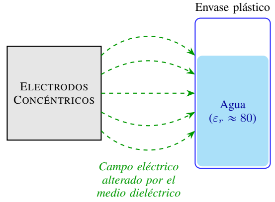
Fig. 5. Interacción del campo eléctrico del sensor capacitivo CR18-8DN con un medio de alta permitividad (agua).
