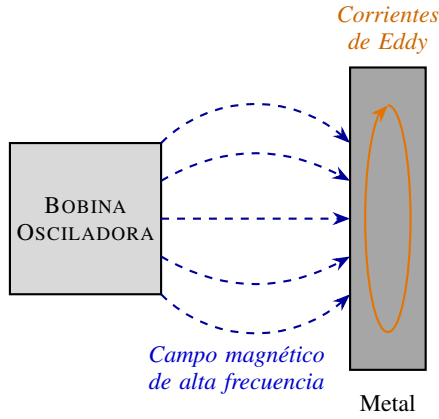
Fig. 3. Principio de inducción electromagnética y generación de corrientes de Foucault en el sensor PR12-4DN.
