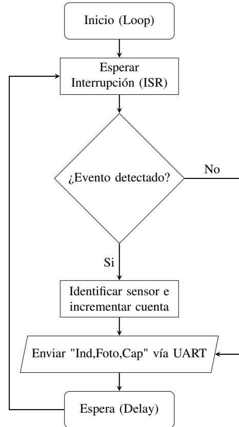
Fig. 8. Diagrama de flujo del firmware de conteo y discriminación implementado en el ESP32.
