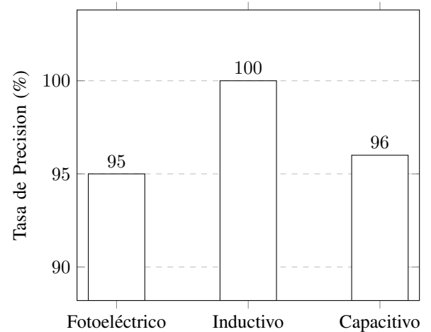
Fig. 11. Tasa de precisión en la detección y clasificación por tipo de sensor tras las pruebas experimentales del lote de producción.
