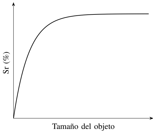
Fig. 4. Relación entre el tamaño del objeto y la distancia de detección relativa ( S_r ) de un sensor inductivo.
