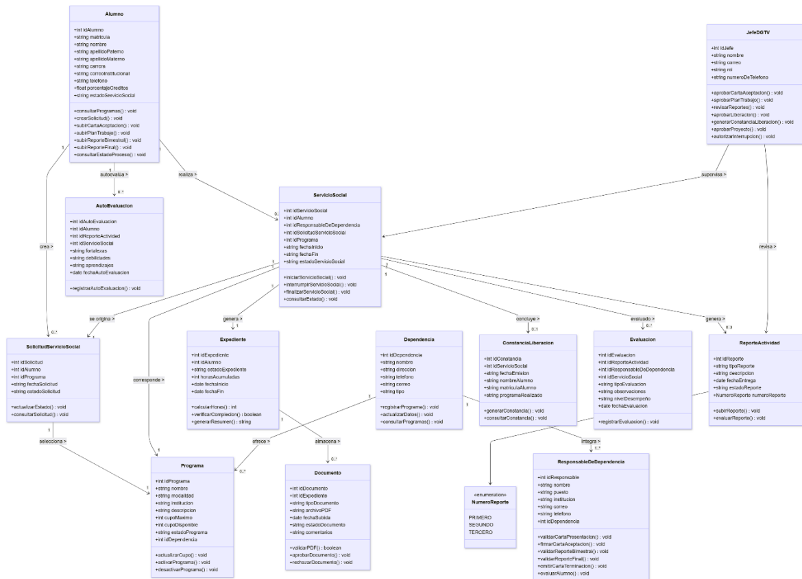
Ilustración 4. Diagrama de clases UML del Sistema de Gestión de Servicio Social del ITChetumal
