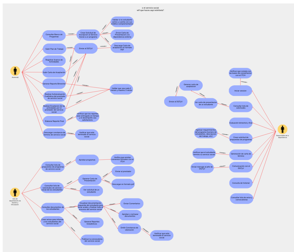
Ilustración 3. Diagrama de casos de uso del Sistema de Gestión de Servicio Social del ITChetumal
