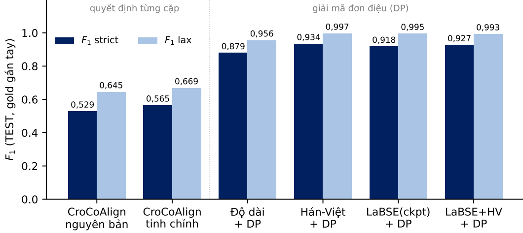
Hình 4: F_1 strict và lax trên TEST của sáu hệ thống (số liệu của Bảng 4). Ranh giới giữa hai nhóm là cách giải mã: quyết định từng cặp độc lập (CroCoAlign) so với quy hoạch động đơn điệu.
