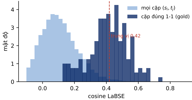
Hình 6: Phân bố cosine LaBSE của 160 cặp một-một trong gold (đậm) so với toàn bộ các cặp (s_i, t_j) của ba mục TEST (nhạt). Hai phân bố tách nhau nhưng cặp đúng chỉ có trung vị 0,42.
