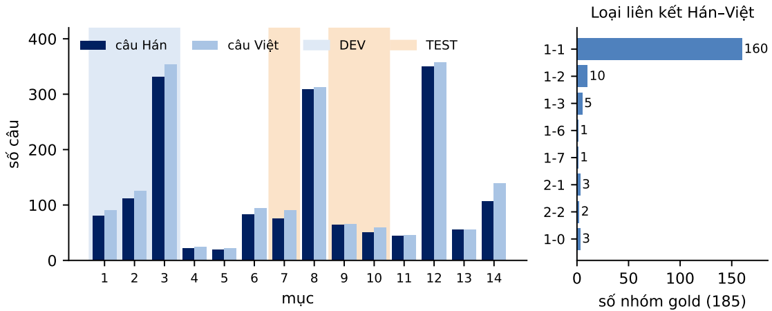
Hình 3: Trái: số câu Hán và câu Việt của 14 mục sau tiền xử lý (mục DEV và TEST được đánh dấu). Phải: phân bố loại liên kết trong 185 nhóm gold gán tay; ngoài 160 nhóm một-một còn có các nhóm một-nhiều dài do chú giải và lời bình.
