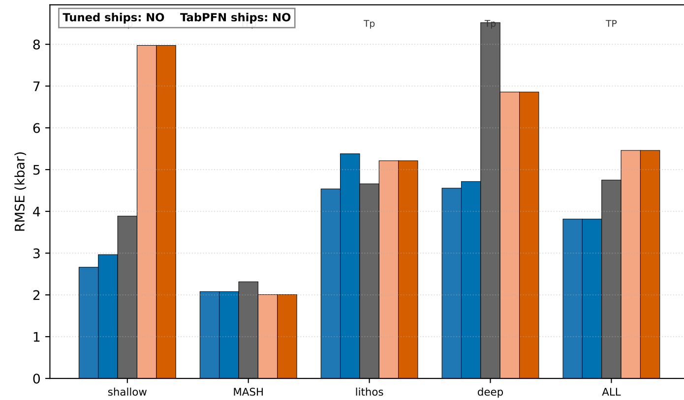
(d) Opx only P (kbar)
