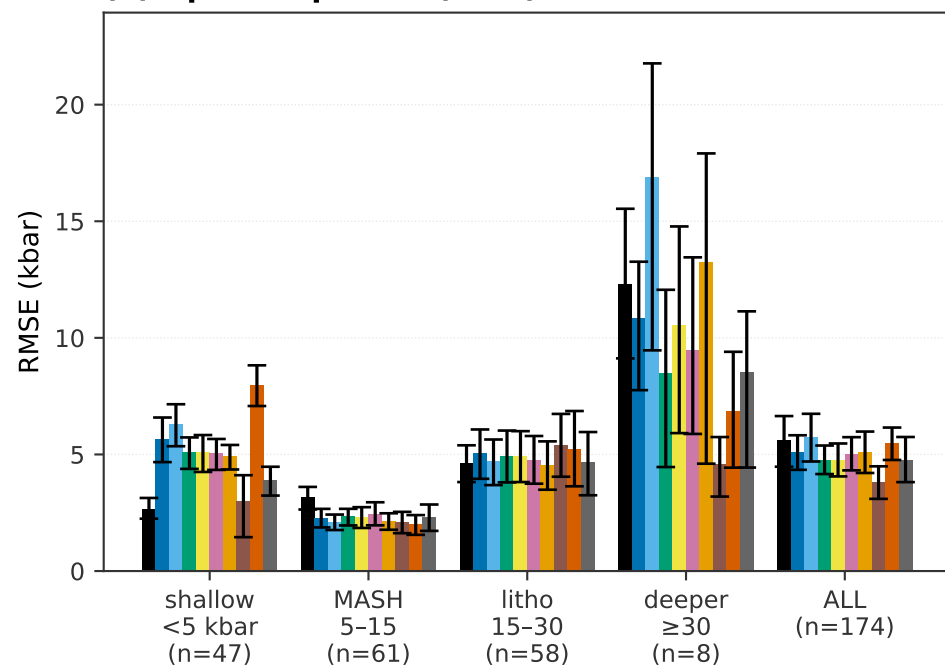
(b) Opx + Liquid · P (kbar)
