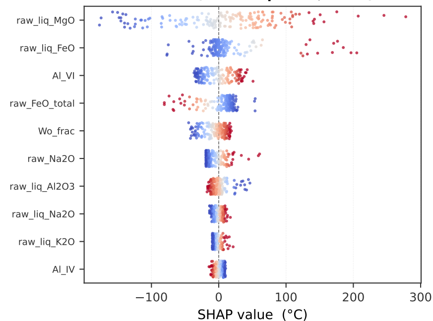
(a) Opx + Liquid · T (°C) ElasticNet/raw (LinearExplainer, exact)
