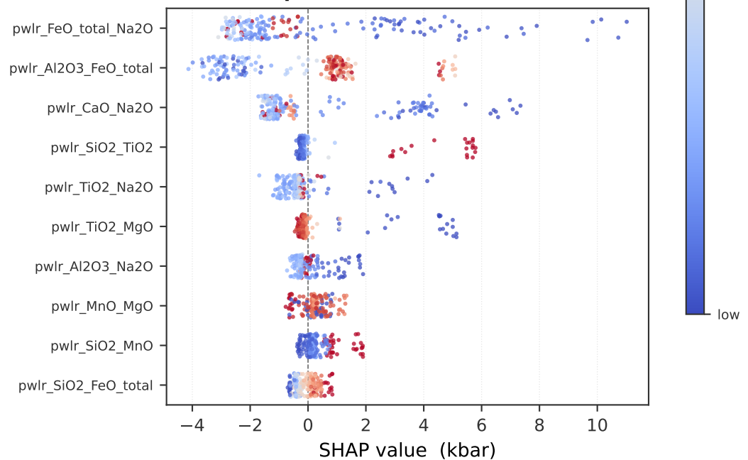
(d) Opx only · P (kbar) shown: RF/pwlr (TabPFN winner has no SHAP)
