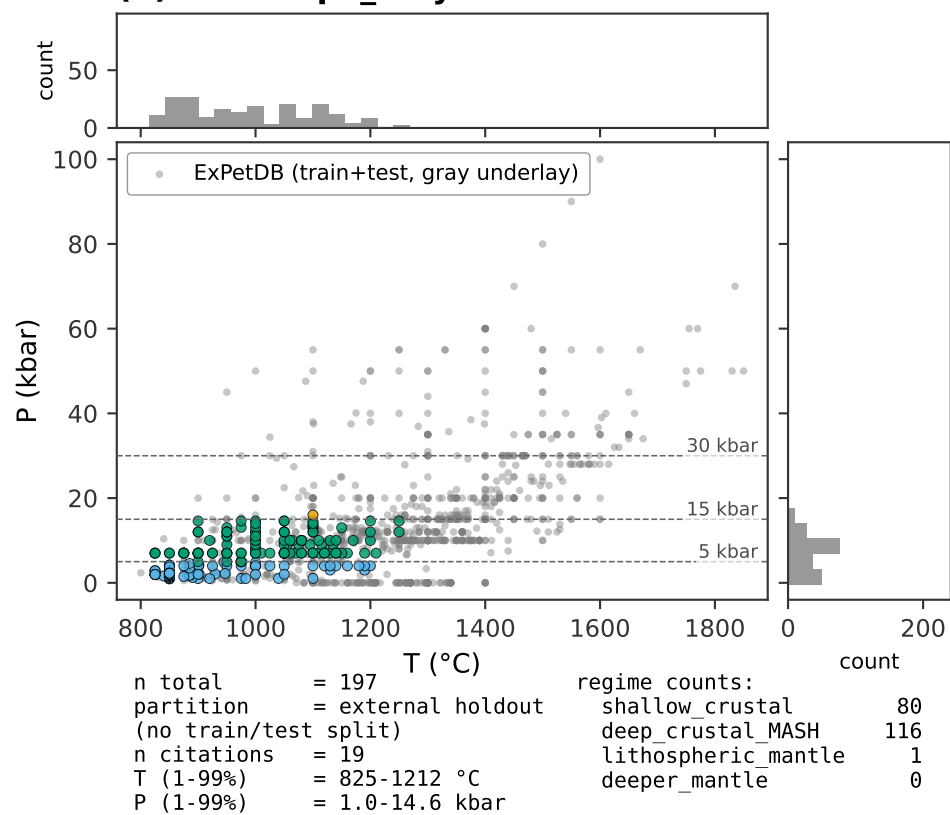
(d) ArcPL opx_only held-out n=197
