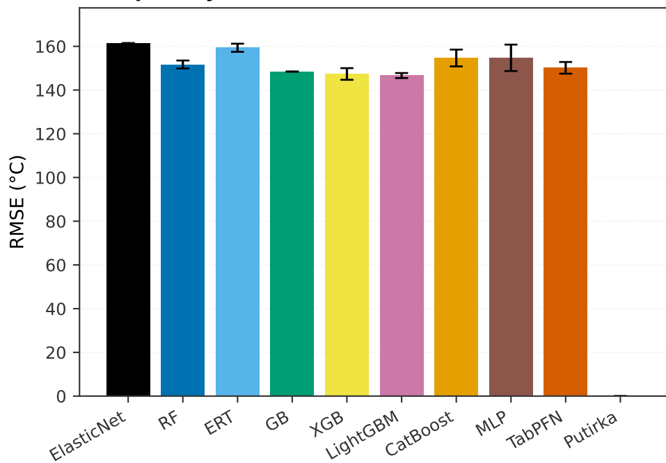
(c) Opx only · T (°C)
