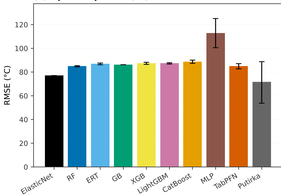
(a) Opx + Liquid · T (°C)
