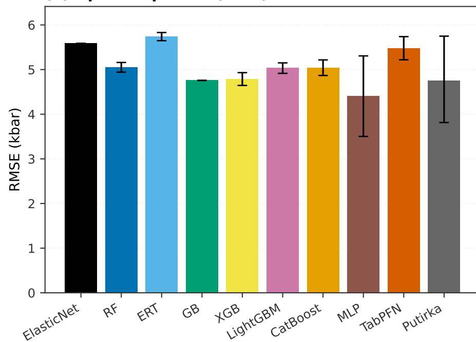
(b) Opx + Liquid · P (kbar)
