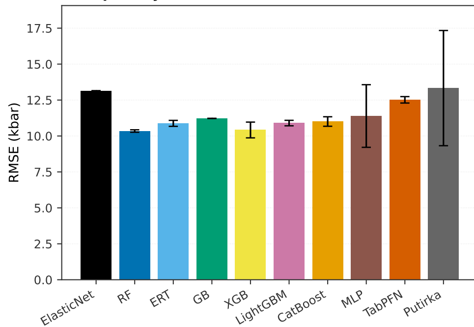
(d) Opx only · P (kbar)
