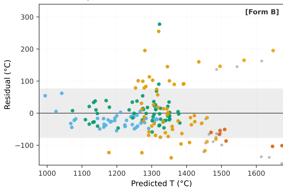
(a) Opx + Liquid · T (°C) ElasticNet/raw
