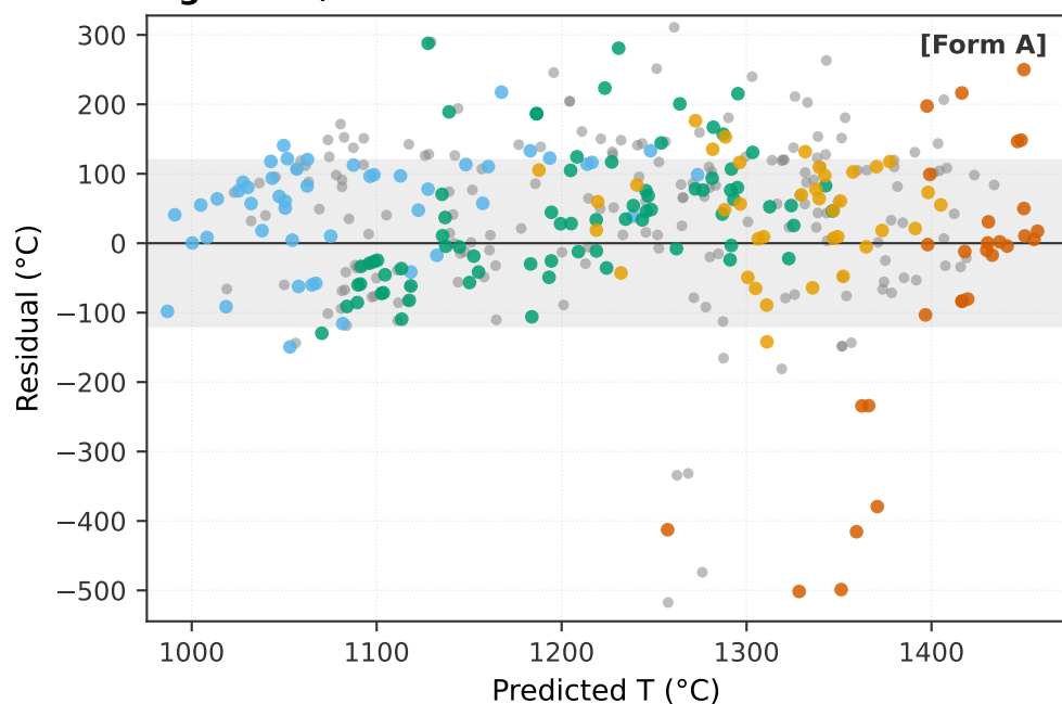
(c) Opx only · T (°C) LightGBM/alr
