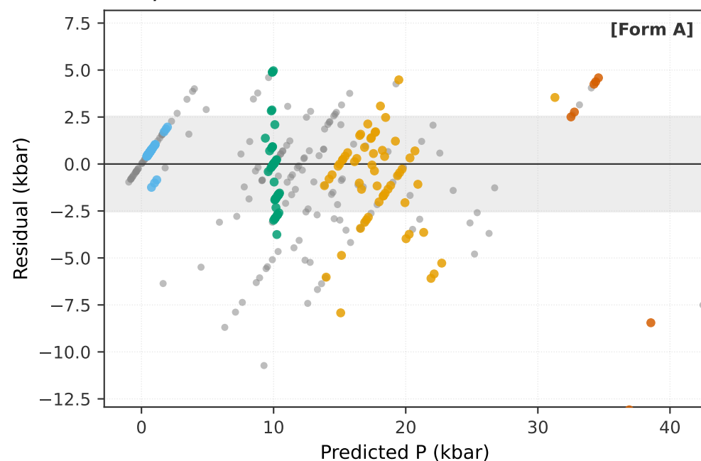
(b) Opx + Liquid · P (kbar) MLP/raw
