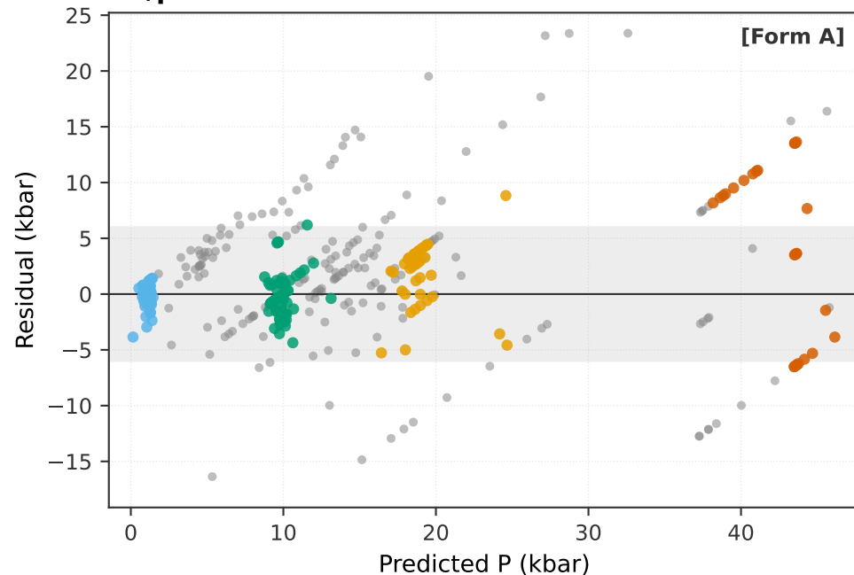
(d) Opx only · P (kbar) RF/pwlr
